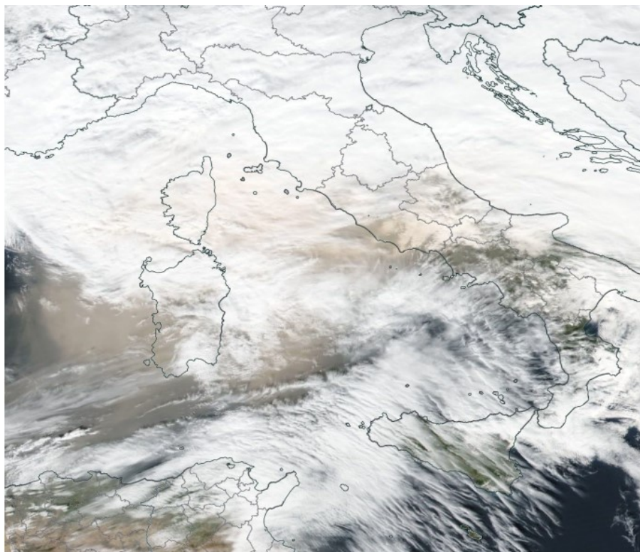
Figura 4. Immagine del Satellite MODIS TERRA elaborazione dust 01 Marzo 2018 ore 10.00 UTC. Fonte NASA.
