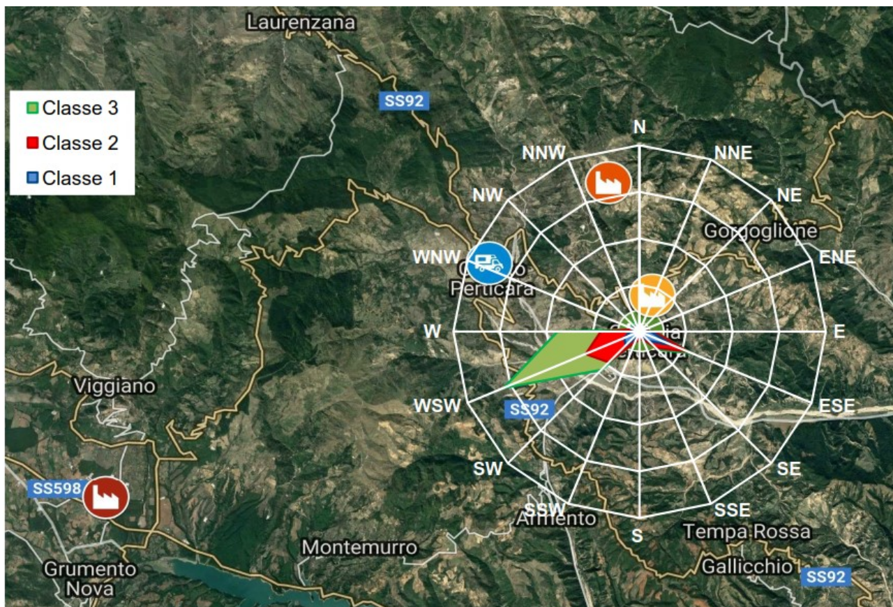
Figura 3. Rosa dei venti (per i valori tabellari si vedano i risultati riportati in seguito. Immagine estratta da Google maps.
