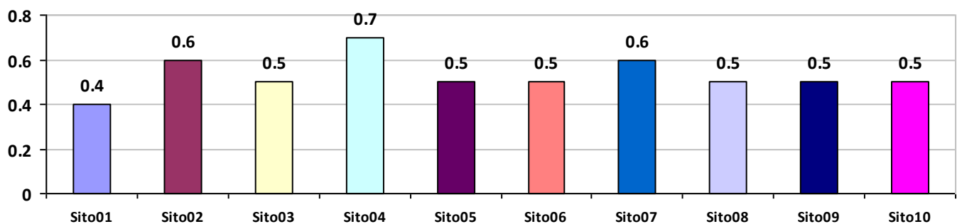
Concentrazioni medie di H2S - Anno 2020
