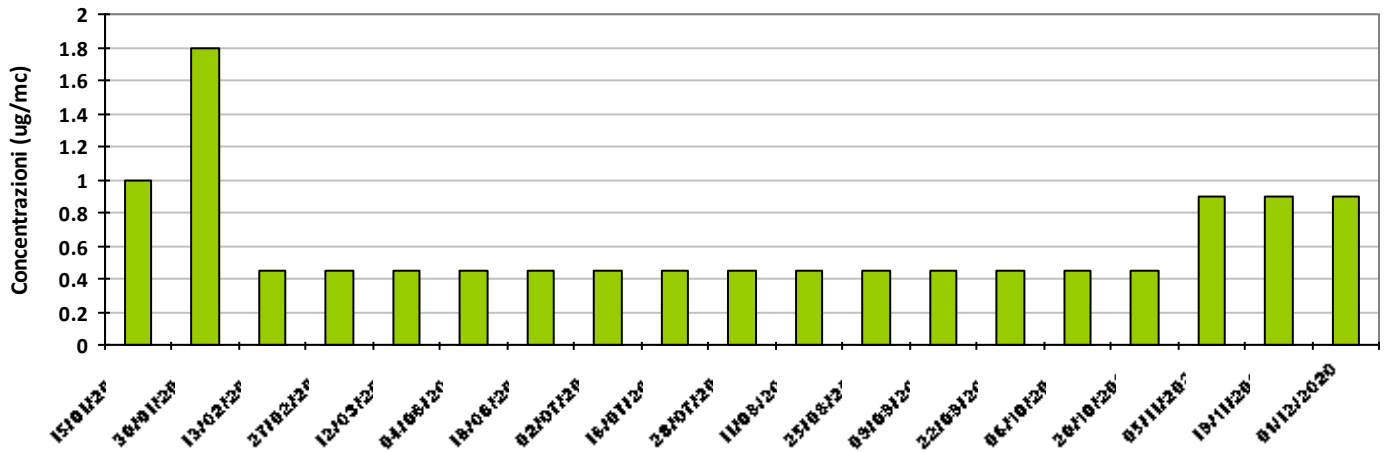
Sito 12 - Diagramma dei valori di concentrazione di H2S rilevati.
