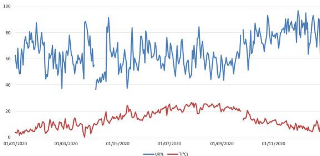
Figura 7.1 - Andamento dell'Umidità relativa (UR) e della Temperatura nel periodo di riferimento – Stazione di Viggiano
