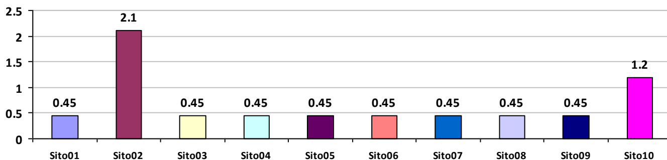
Concentrazioni Massime di H 2 S - Anno 2020
