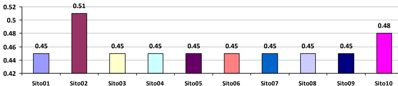
Concentrazioni medie di H 2 S - Anno 2020
