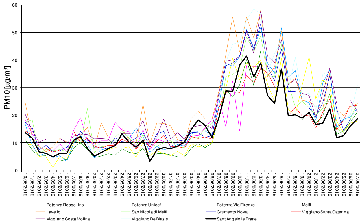
Figura 6. Valori di PM10 giornalieri rilevati dalla rete di qualità dell'aria regionale. I valori riportati per Sant'Angelo le Fratte sono quelli medi giornalieri rilevati mediante contaparticelle ottico GRIMM EDM 180.
