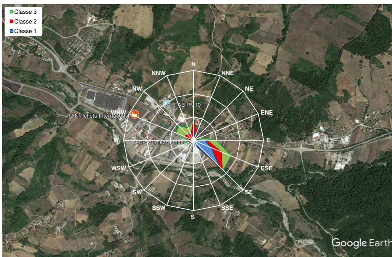
Figura 4. Rosa dei venti (per i valori tabellari si vedano i risultati riportati in seguito). Immagine estratta da Google maps.
