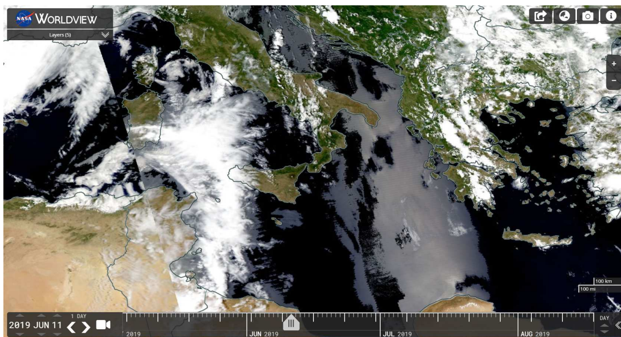
Figura 5. Immagine del Satellite MODIS AQUA del 11/06/2019. Fonte NASA.
