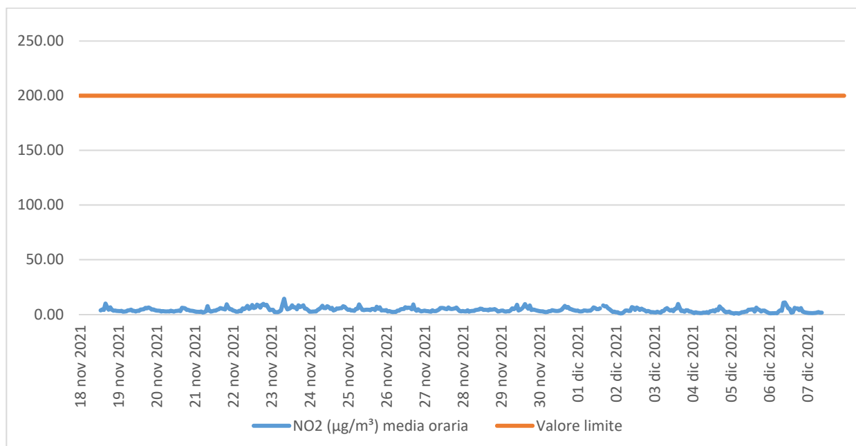
Figura 8.1 - Concentrazione (µg/m 3 ) media oraria di NO 2 .
