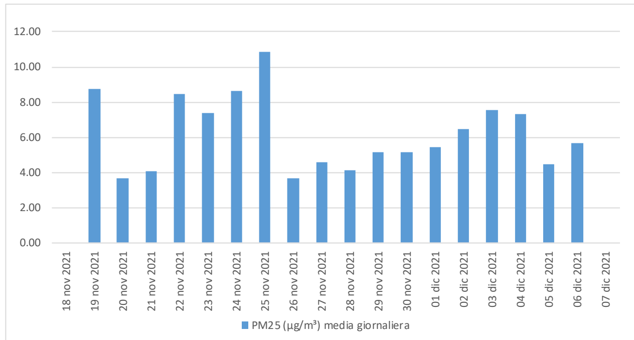
Figura 10.1 - Concentrazione ( \mu\text{g}/\text{m}^3 ) media giornaliera di PM2.5.
