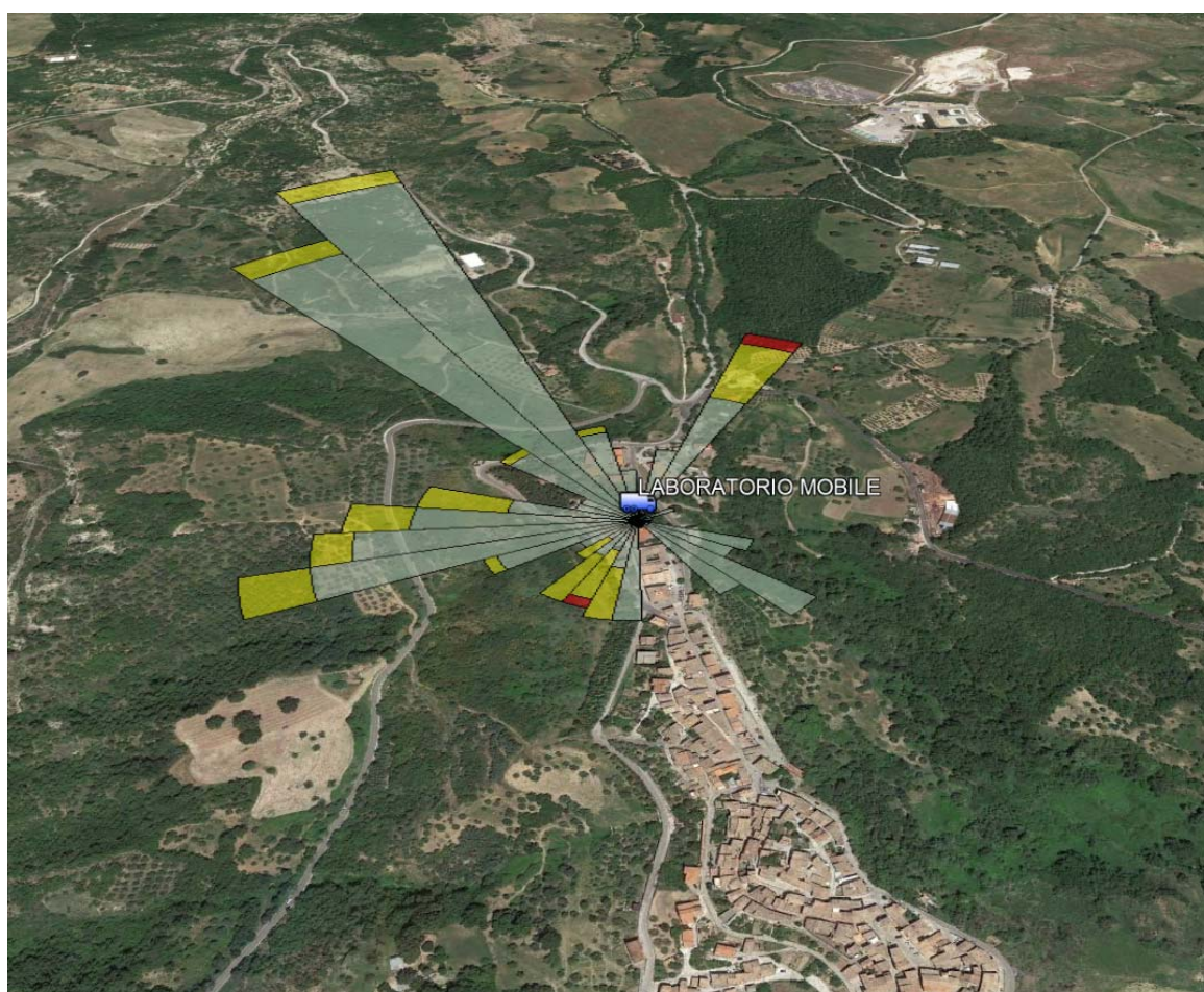
Figura 12.8 - Rosa dei venti su base ortofoto.
