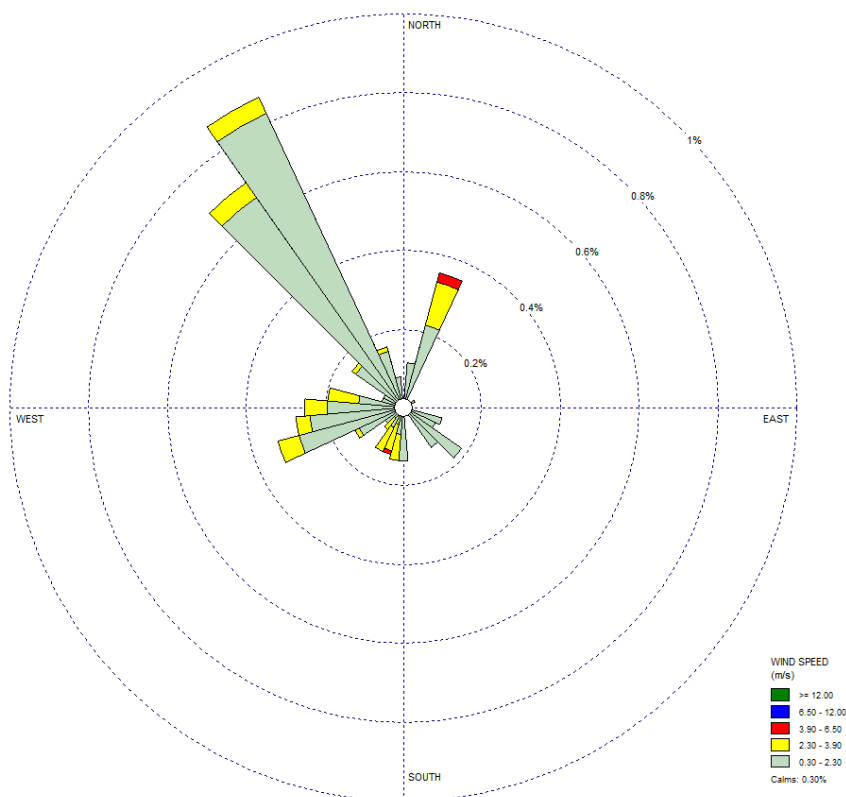
Figura 12.9 - Rosa dei venti - Media del periodo.
