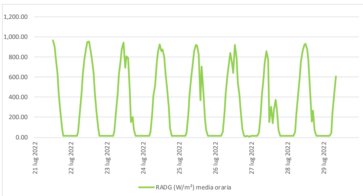
Figura 12.4 - Radiazione solare.
