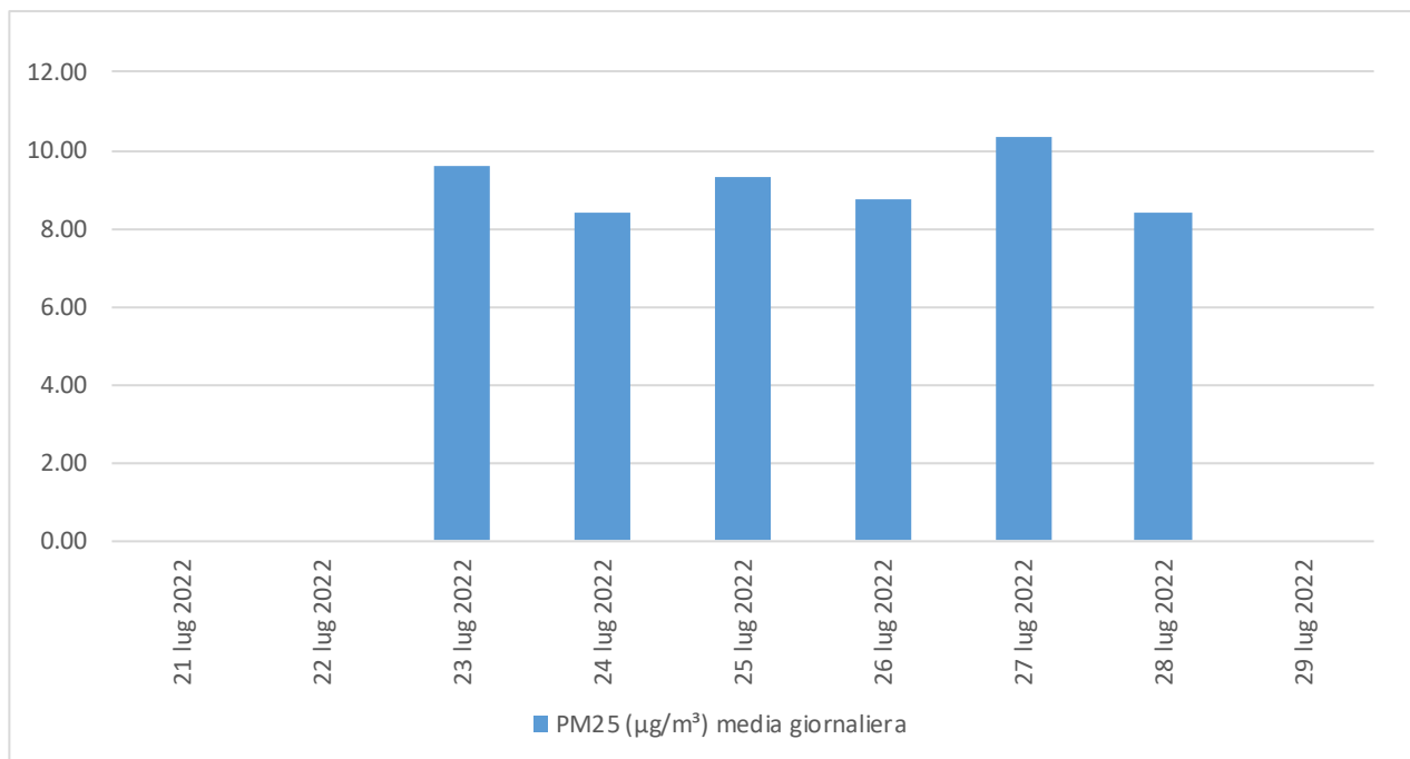
Figura 10.2 - Concentrazione (µg/m³) media giornaliera di PM2.5.
