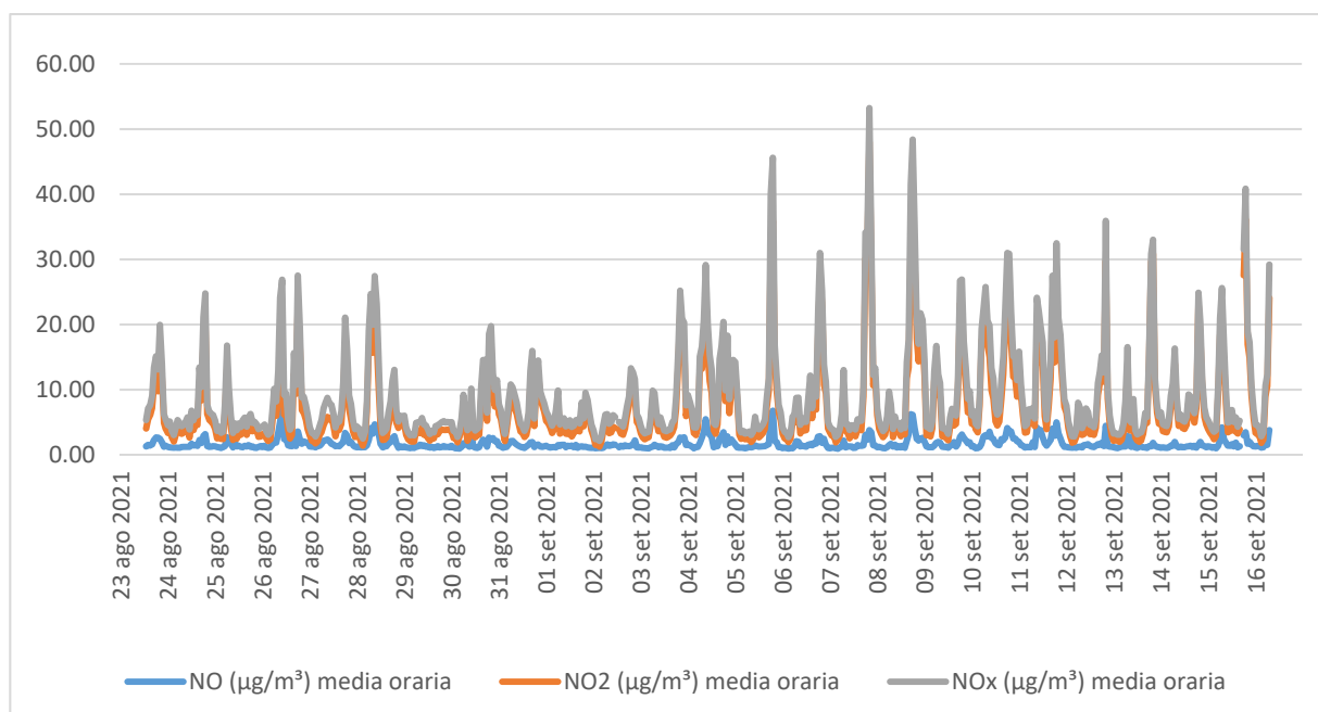
Figura 8.2 - Concentrazione ( \mu\text{g}/\text{m}^3 ) media oraria di Ossidi di azoto rapportati al valore limite di norma.
