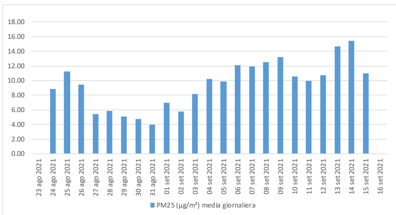
Figura 10.1 - Concentrazione (µg/m³) media giornaliera di PM2.5.
