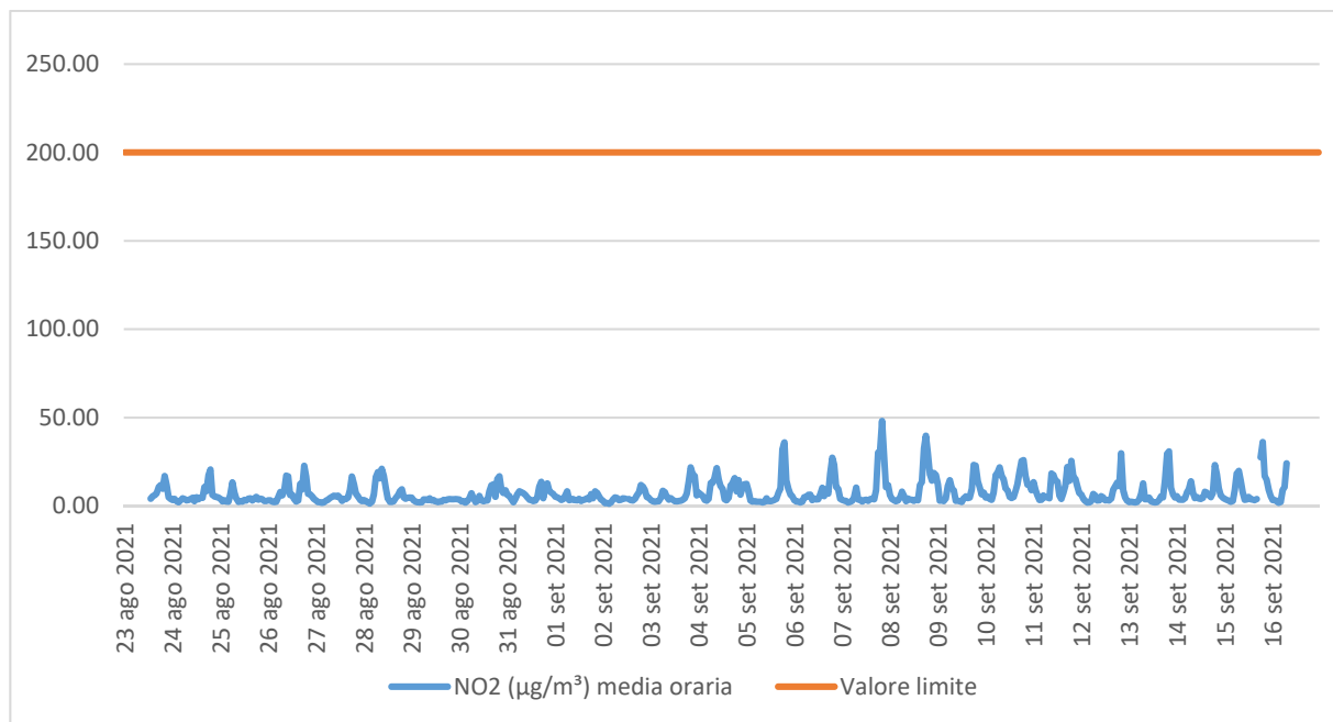
Figura 8.1 - Concentrazione ( \mu\text{g}/\text{m}^3 ) media oraria di NO2.
