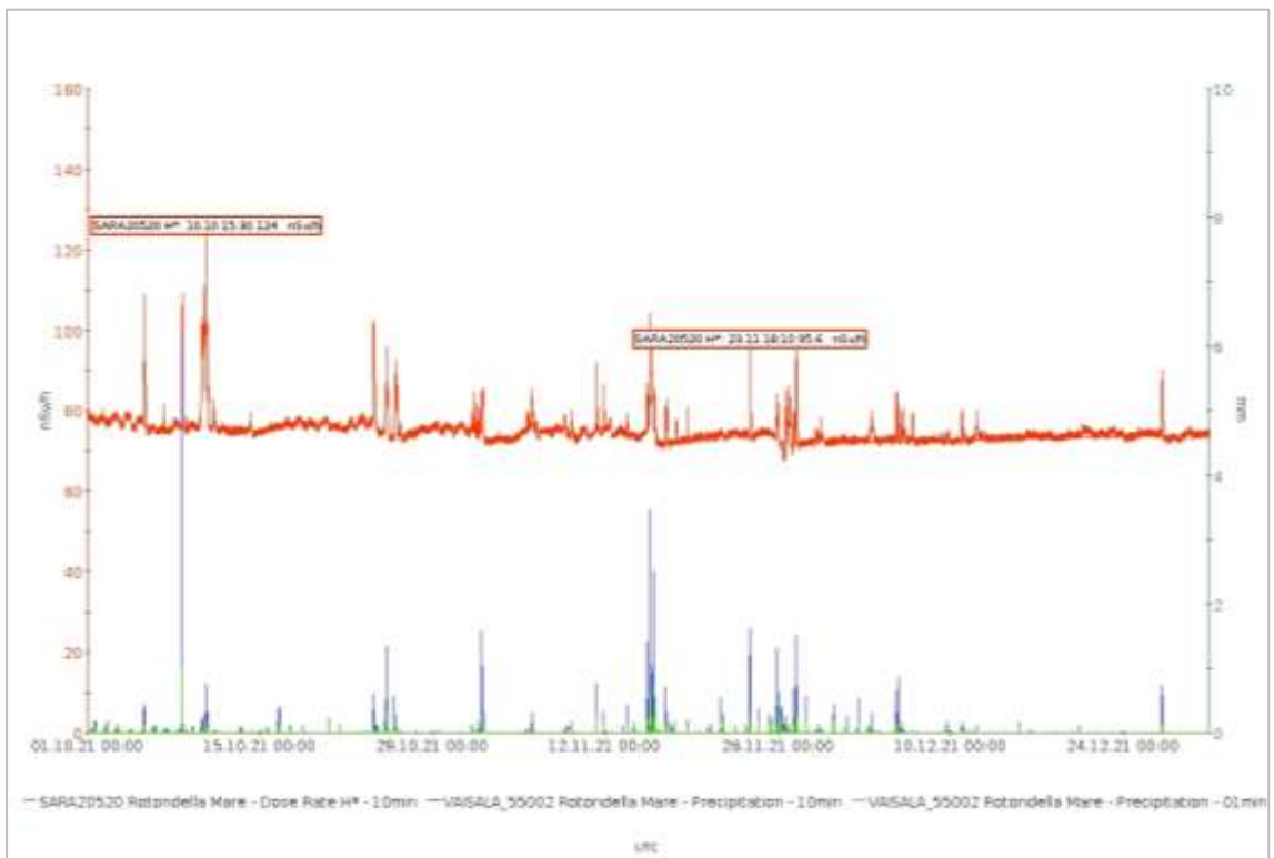
Figura 2.2.2 – Stazione di Rotondella Mare: grafico delle misurazioni del IV trimestre 2021
