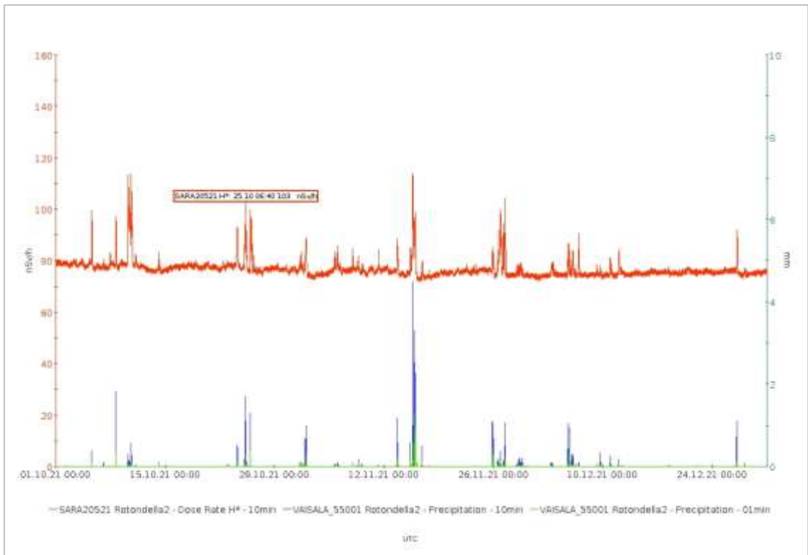
Figura 2.2.1 – Stazione di Rotondella 2: grafico delle misurazioni del IV trimestre 2021
