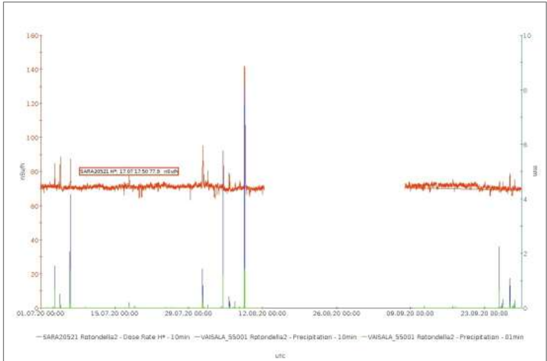
Figura 2.2.1 – Stazione di Rotondella 2: grafico delle misurazioni del III trimestre 2020
