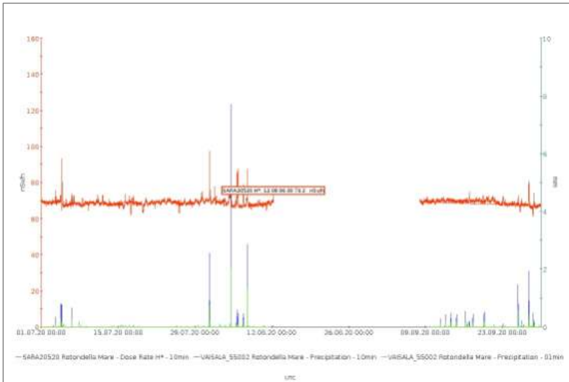
Figura 2.2.2 – Stazione di Rotondella Mare: grafico delle misurazioni del III trimestre 2020
