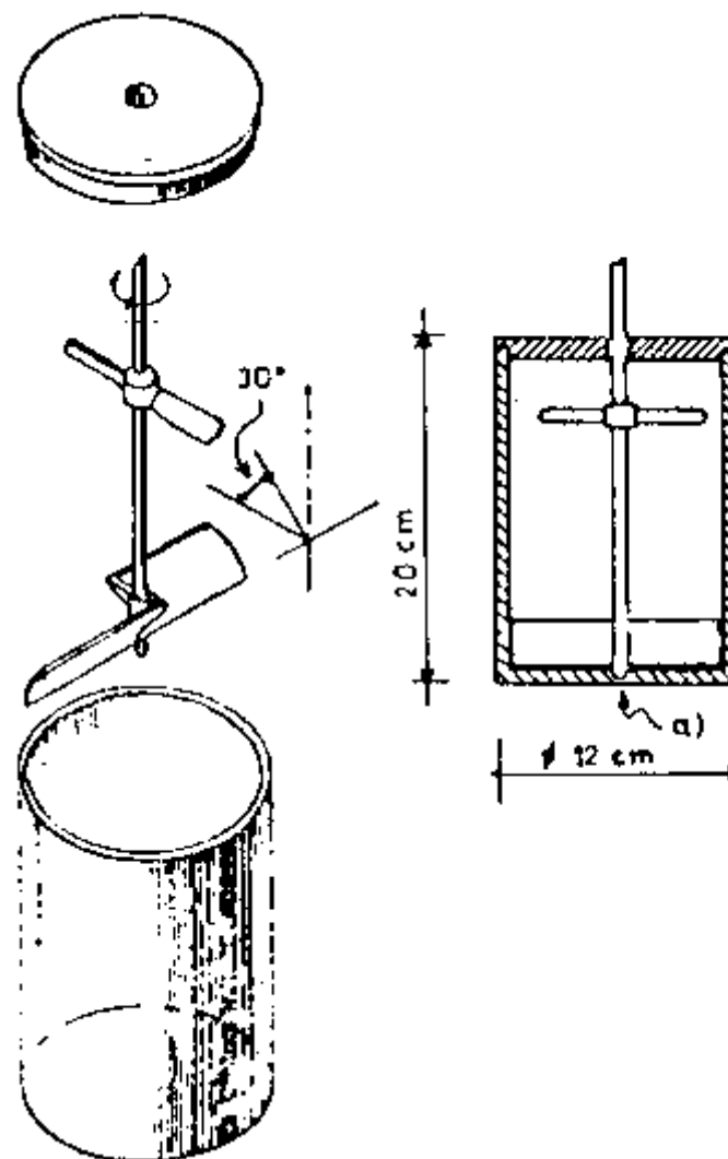
Figura 1 - Estrattore
