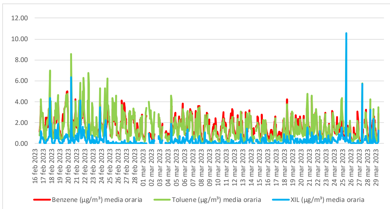
Figura 5.16 - Concentrazione ( \mu\text{g}/\text{m}^3 ) media oraria di BTX.
