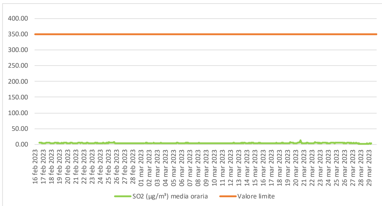
Figura 5.3 - Concentrazione ( \mu\text{g}/\text{m}^3 ) media oraria di SO 2 .
