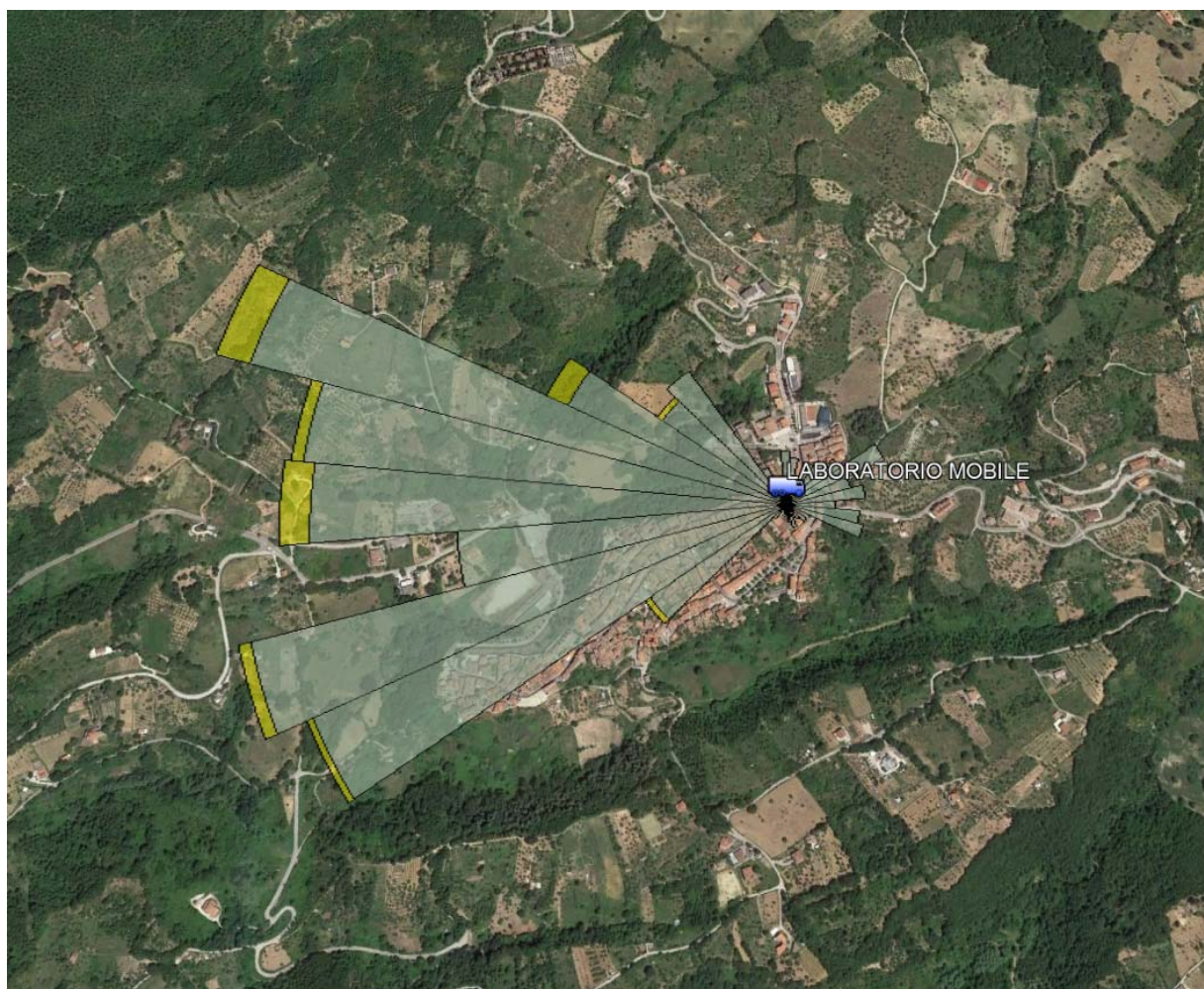
Figura 6.8 - Rosa dei venti su base ortofoto
