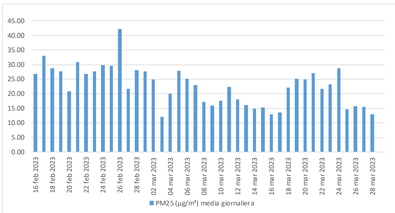
Figura 5.14 - Concentrazione (µg/m³) media giornaliera di PM2.5.
