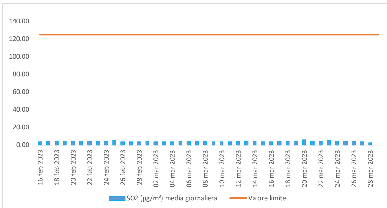
Figura 5.4 - Concentrazione ( \mu\text{g}/\text{m}^3 ) media giornaliera di SO 2 .
