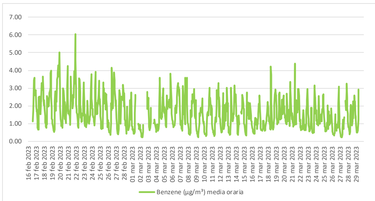
Figura 5.15 - Concentrazione ( \mu\text{g}/\text{m}^3 ) media oraria di Benzene.
