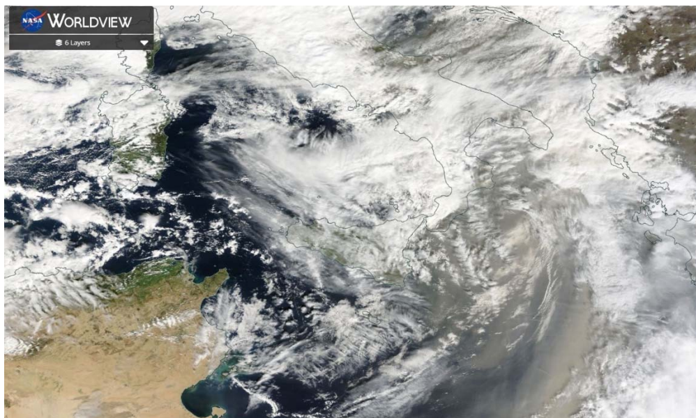
Figura 5.11 - Immagine satellitare dell'intrusione sahariana nel Mediterraneo per il giorno 25 Febbraio 2023 ( https://worldview.earthdata.nasa.gov )
