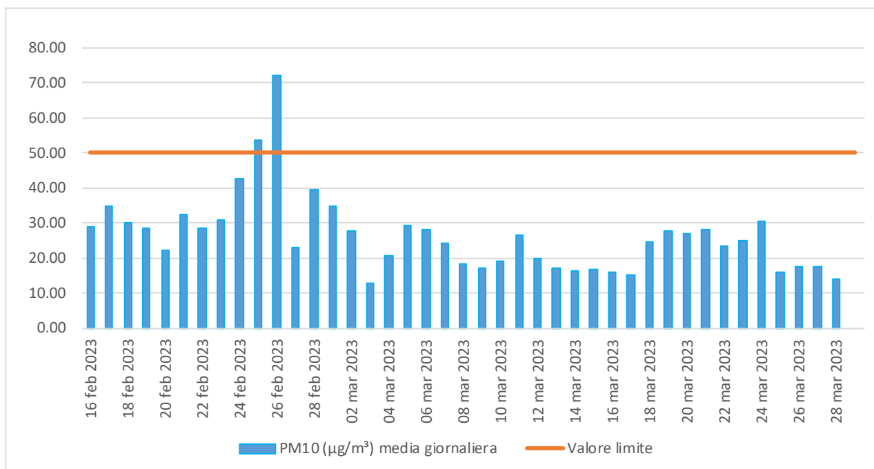
Figura 5.13 - Concentrazione (µg/m³) media giornaliera di PM10.
