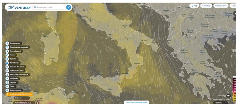
Figura 5.12 - Immagine modellistica del PM10 nel Mediterraneo per il giorno 25 Febbraio 2023 ( https://www.ventusky.com ).
