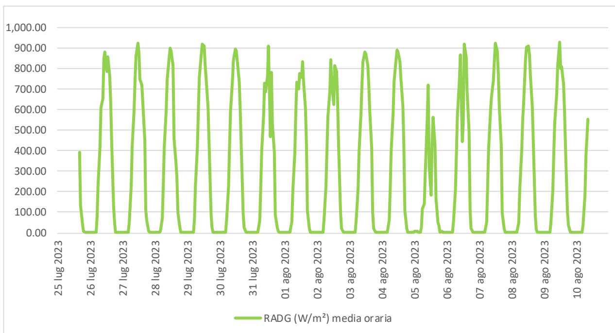
Figura 6.4 - Radiazione Solare.
