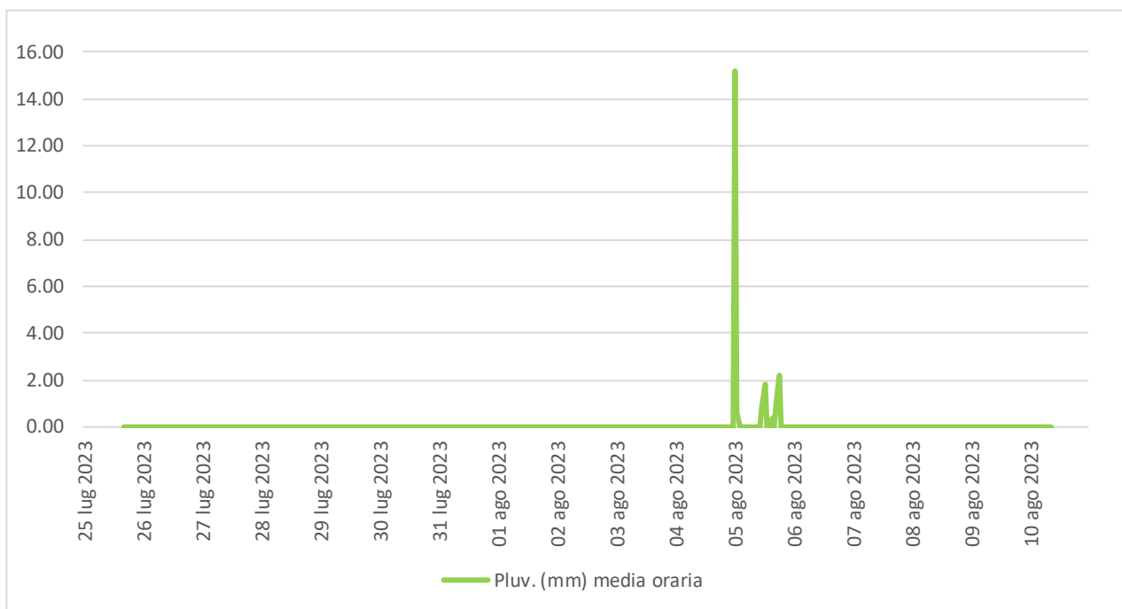
Figura 6.7 - Precipitazioni.
