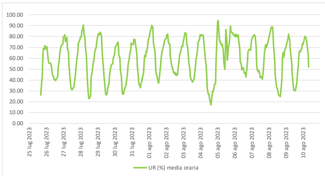
Figura 6.6 - Umidità Relativa.
