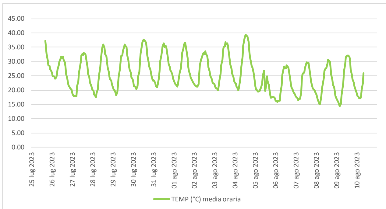
Figura 6.5 - Temperatura.
