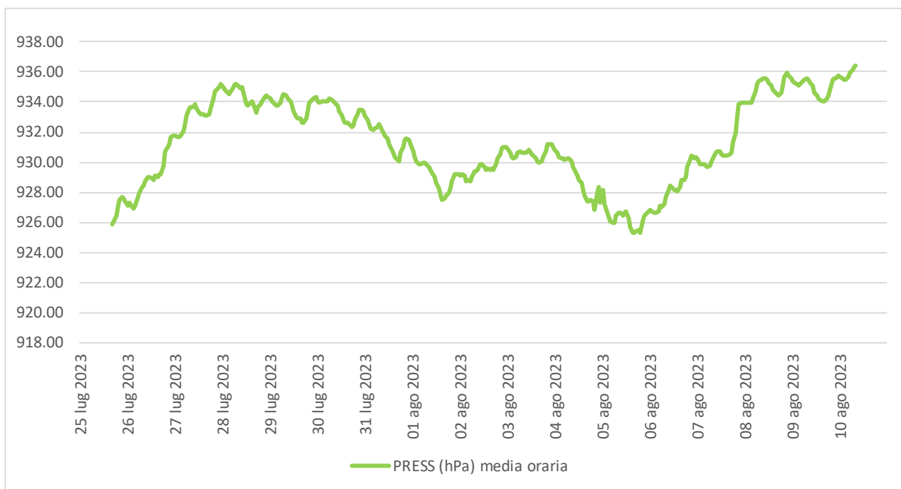
Figura 6.3 - Pressione atmosferica.
