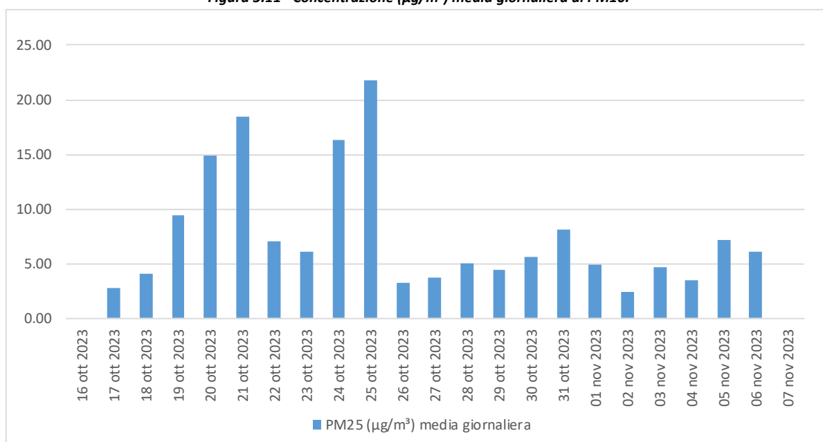
Figura 5.12 - Concentrazione ( \mu\text{g}/\text{m}^3 ) media giornaliera di PM2.5.
