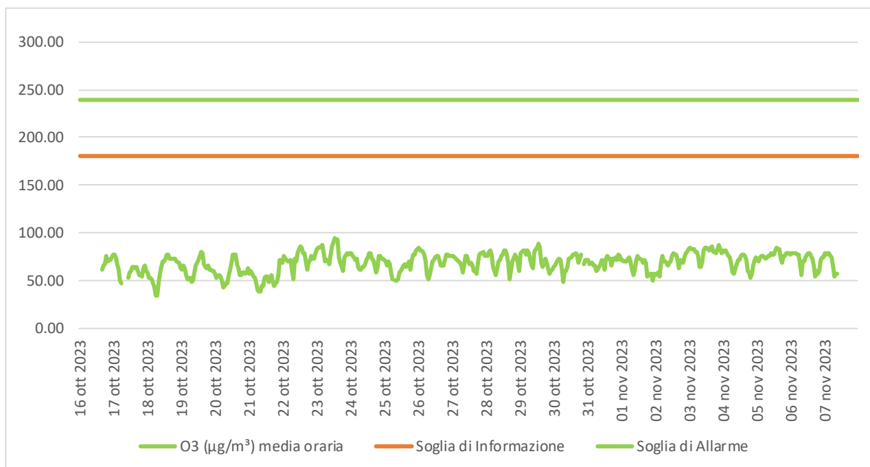
Figura 5.9 - Concentrazione (µg/m³) media oraria di O3.
