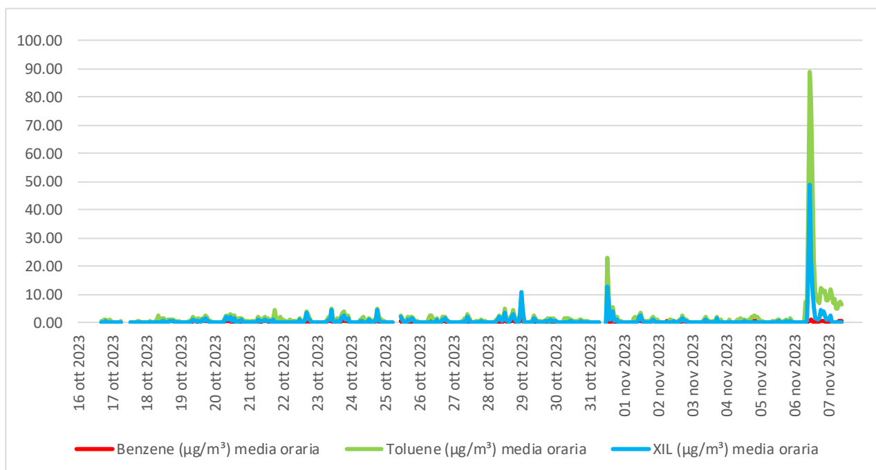
Figura 5.14 - Concentrazione ( \mu\text{g}/\text{m}^3 ) media oraria di BTX.
