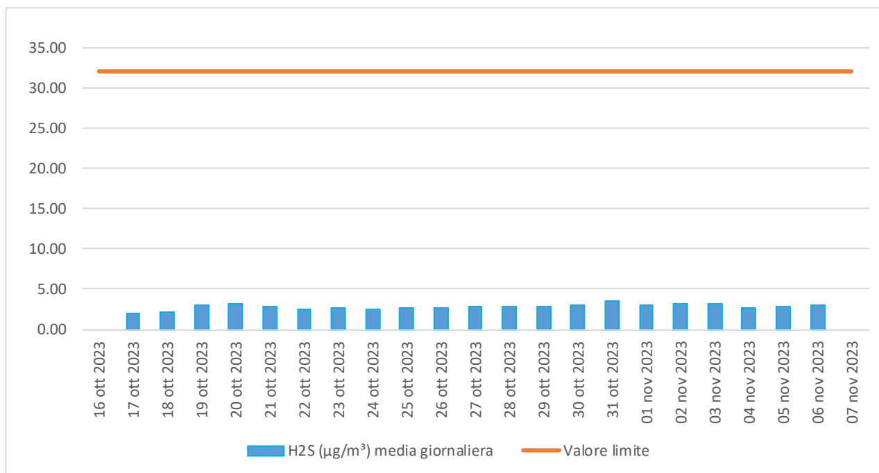
Figura 5.6 - Concentrazione (µg/m 3 ) media giornaliera di H 2 S.
