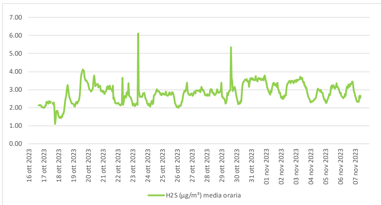
Figura 5.5 - Concentrazione (µg/m 3 ) media oraria di H 2 S.
