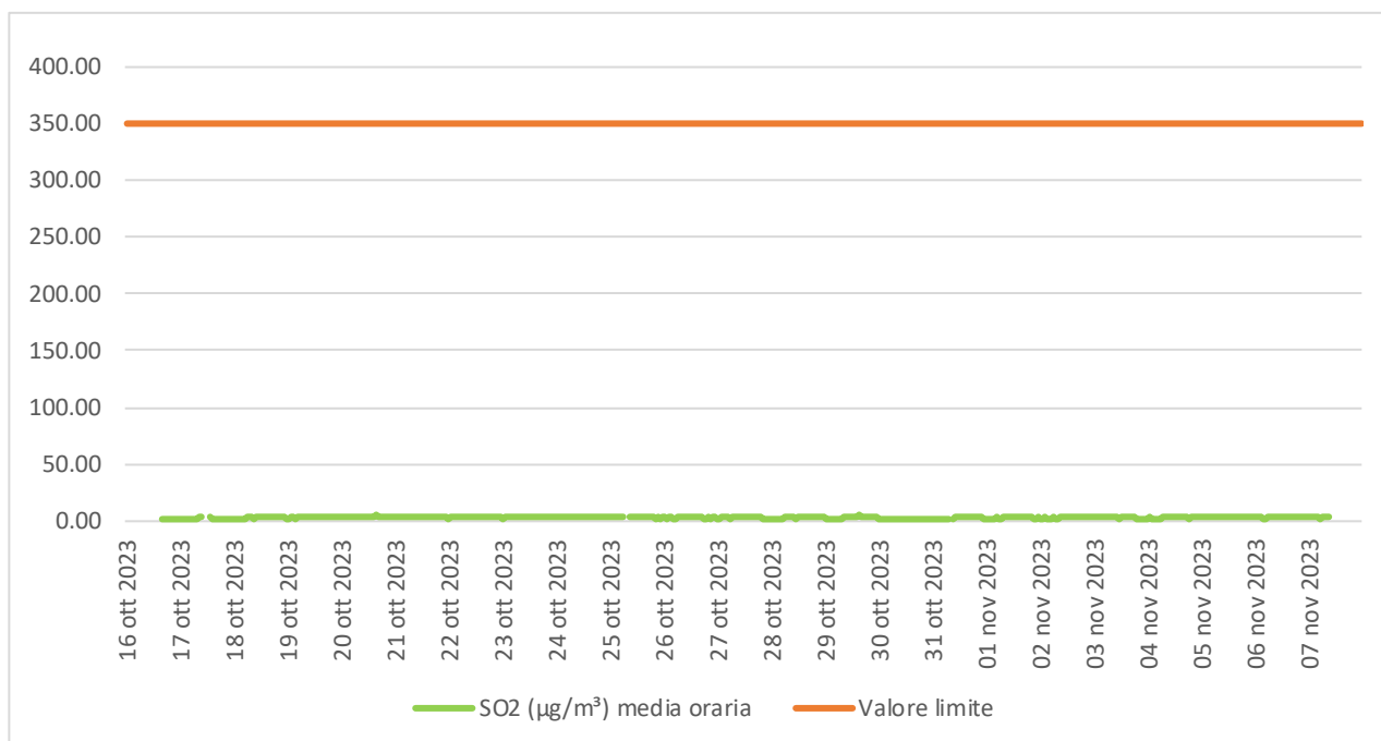
Figura 5.3 - Concentrazione (µg/m³) media oraria di SO2.
