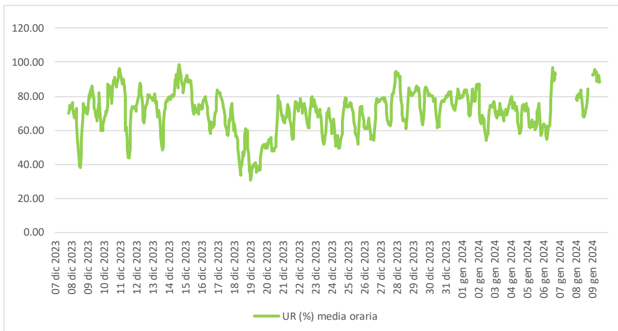
Figura 6.6 - Umidità Relativa.
