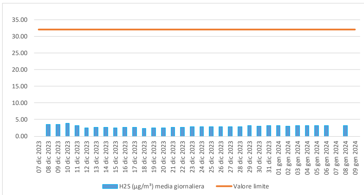
Figura 5.6 - Concentrazione ( \mu\text{g}/\text{m}^3 ) media giornaliera di H2S.
