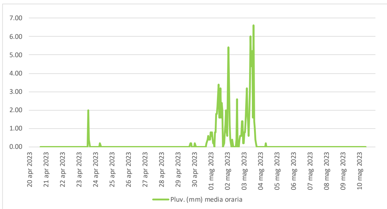
Figura 6.7 - Precipitazioni.
