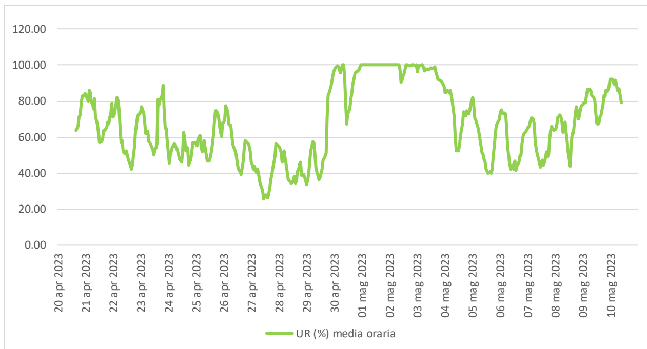
Figura 6.6 - Umidità Relativa.
