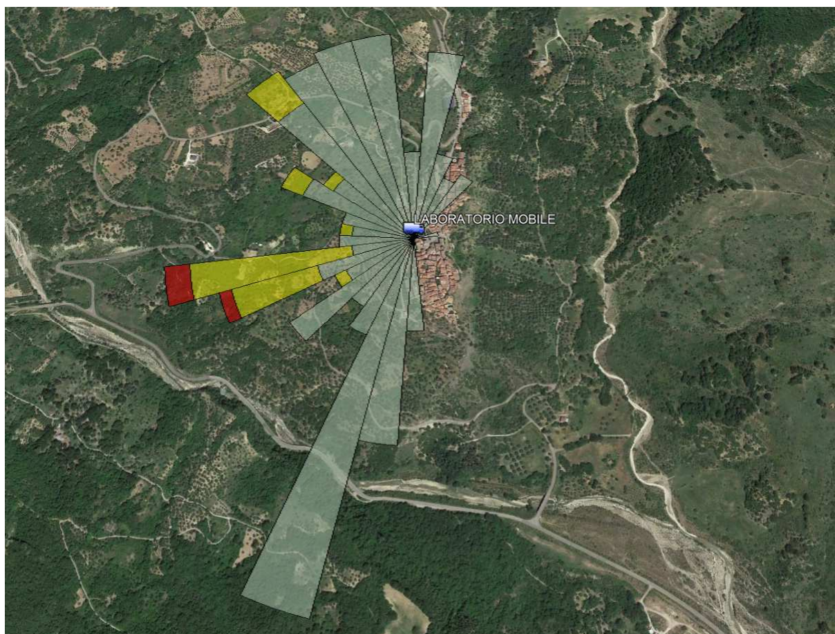
Figura 6.7 - Precipitazioni.
