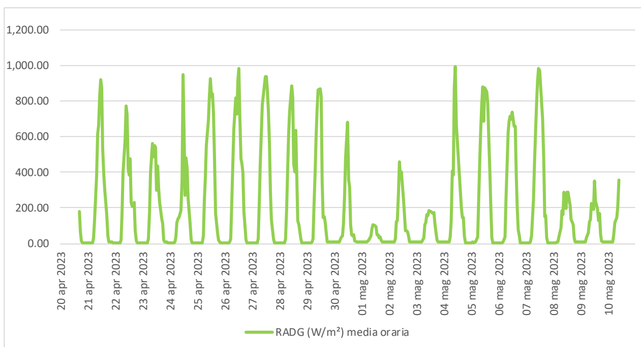
Figura 6.4 - Radiazione Solare.
