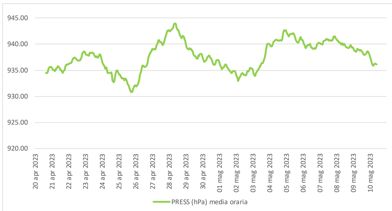
Figura 6.3 - Pressione atmosferica.
