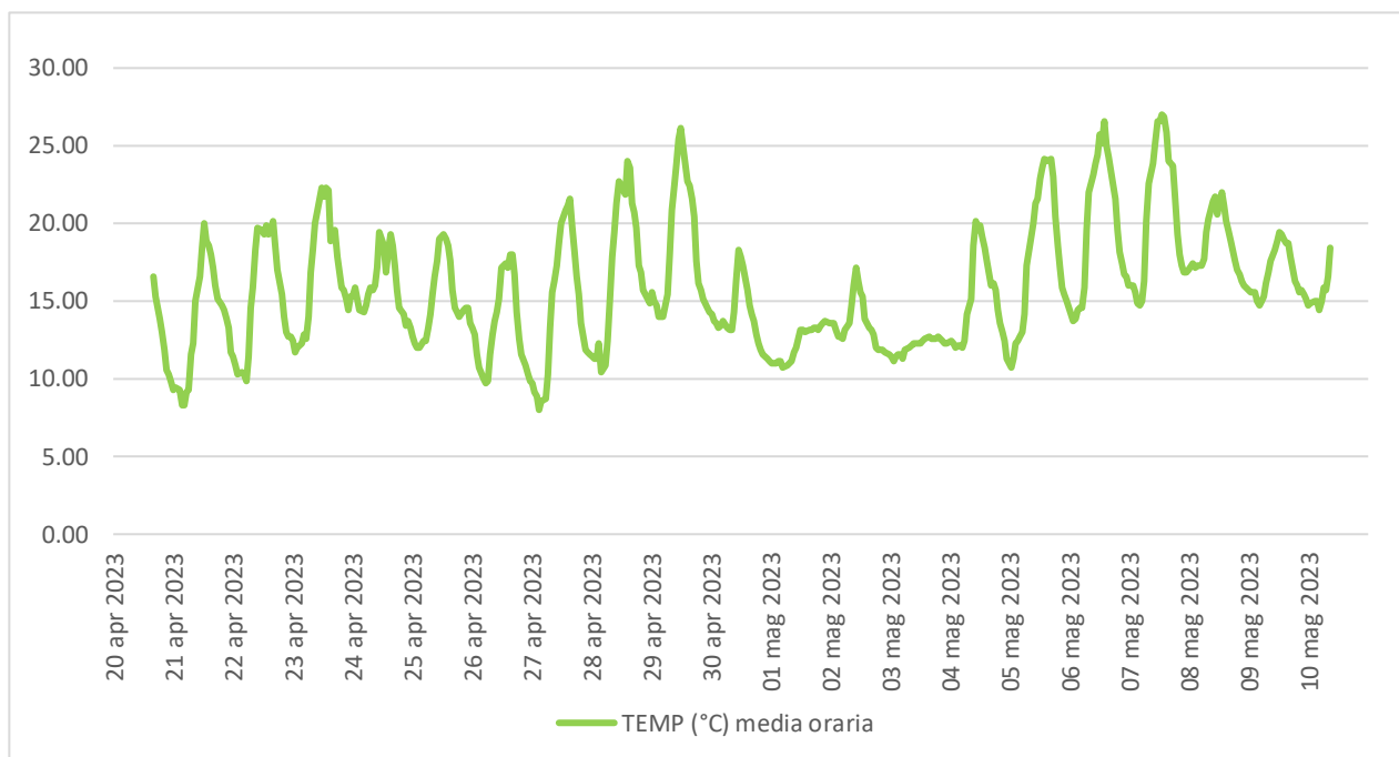
Figura 6.5 - Temperatura.
