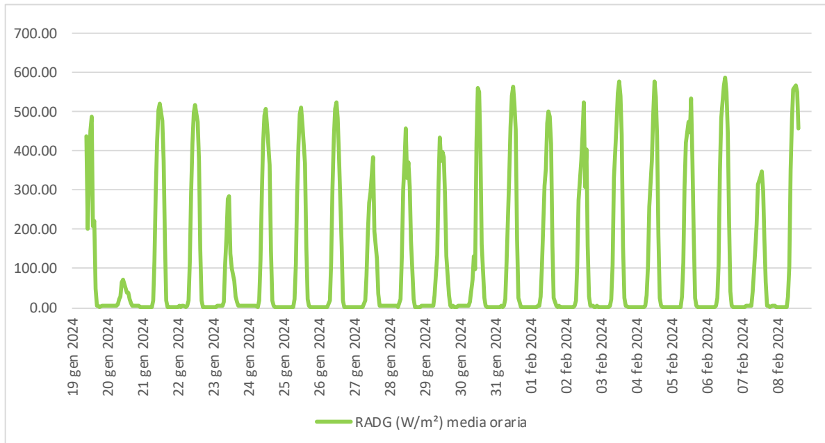
Figura 6.4 - Radiazione Solare.
