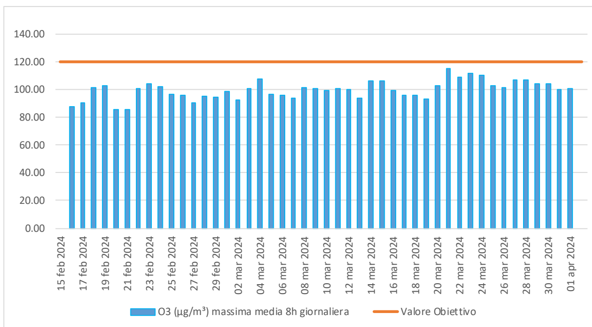
Figura 5.10 - Concentrazione (µg/m 3 ) media mobile sulle 8 ore di O 3 .
