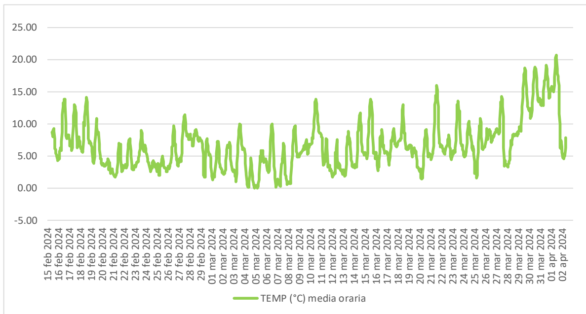
Figura 6.5 - Temperatura.
