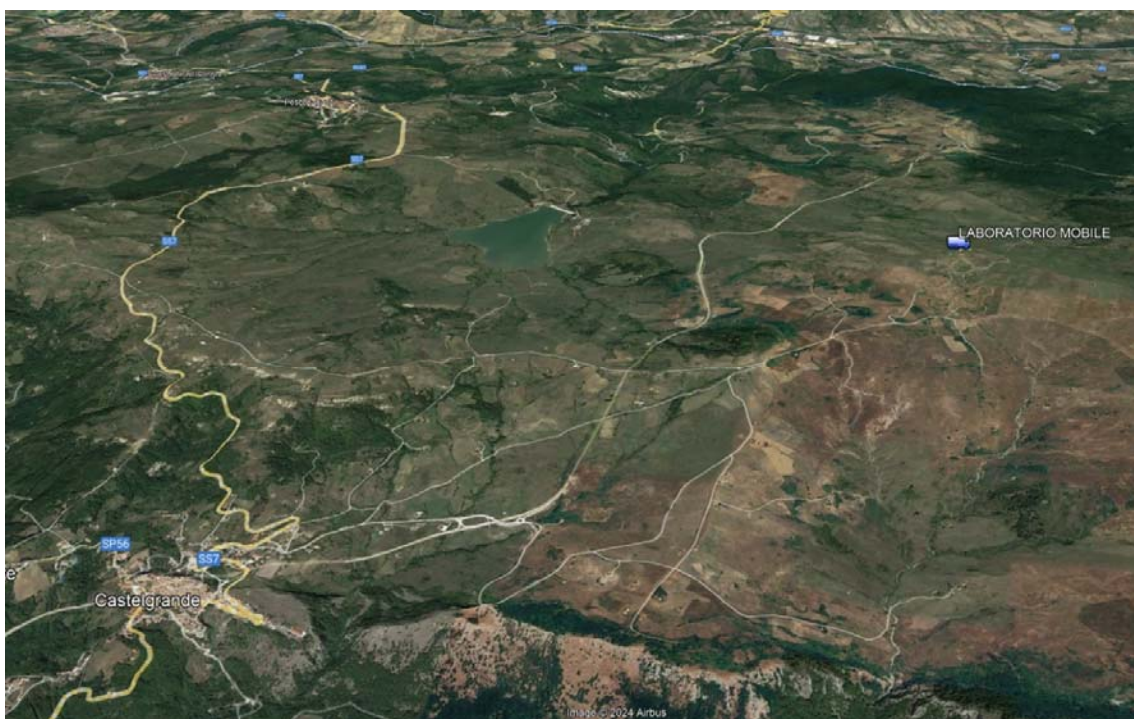
Figura 2.2 - Dettaglio Posizione del Laboratorio Mobile su base ortofoto - Google Earth.
