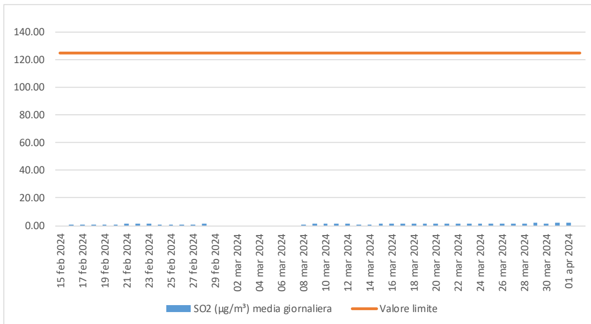
Figura 5.4 - Concentrazione ( \mu\text{g}/\text{m}^3 ) media giornaliera di SO 2 .
