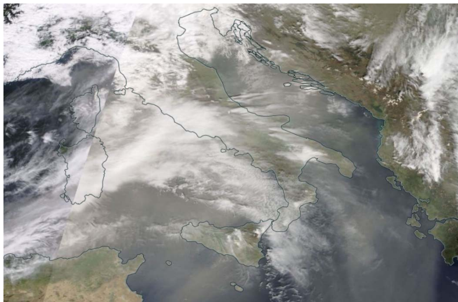
Figura 5.11 - Immagine satellitare dell'intrusione sahariana nel Mediterraneo per il giorno 31 Marzo 2024 ( https://worldview.earthdata.nasa.gov )
