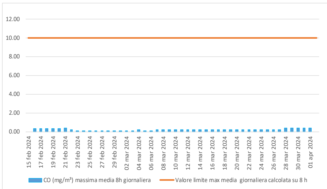
Figura 5.2 - Concentrazione (mg/m³) massima media giornaliera sulle 8 ore di CO.
