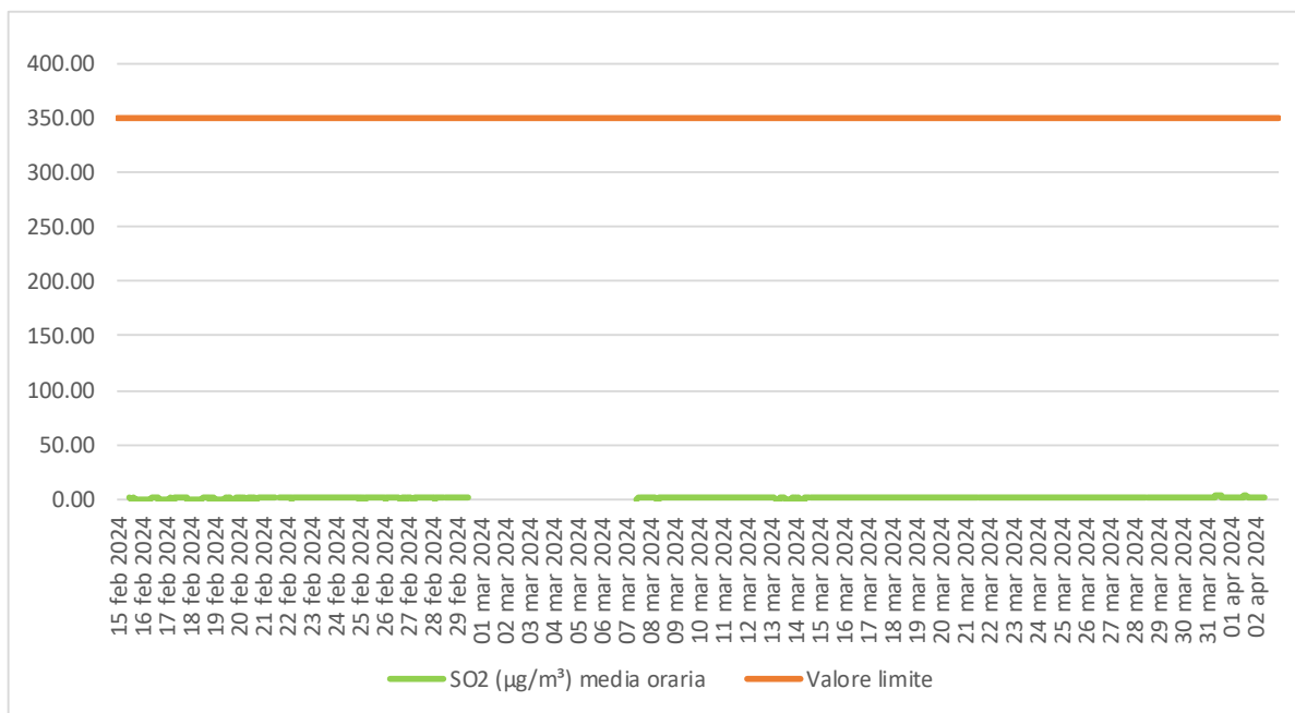
Figura 5.3 - Concentrazione ( \mu\text{g}/\text{m}^3 ) media oraria di SO 2 .
