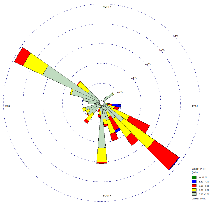
Figura 6.9 - Rosa dei venti - Media del periodo.
