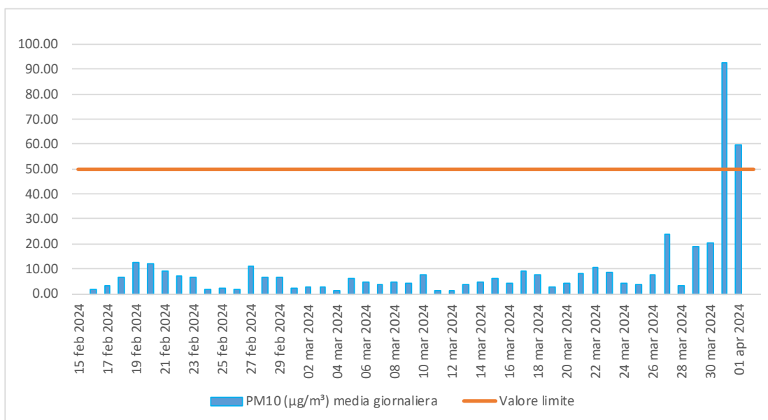
Figura 5.13 - Concentrazione (µg/m³) media giornaliera di PM10.
