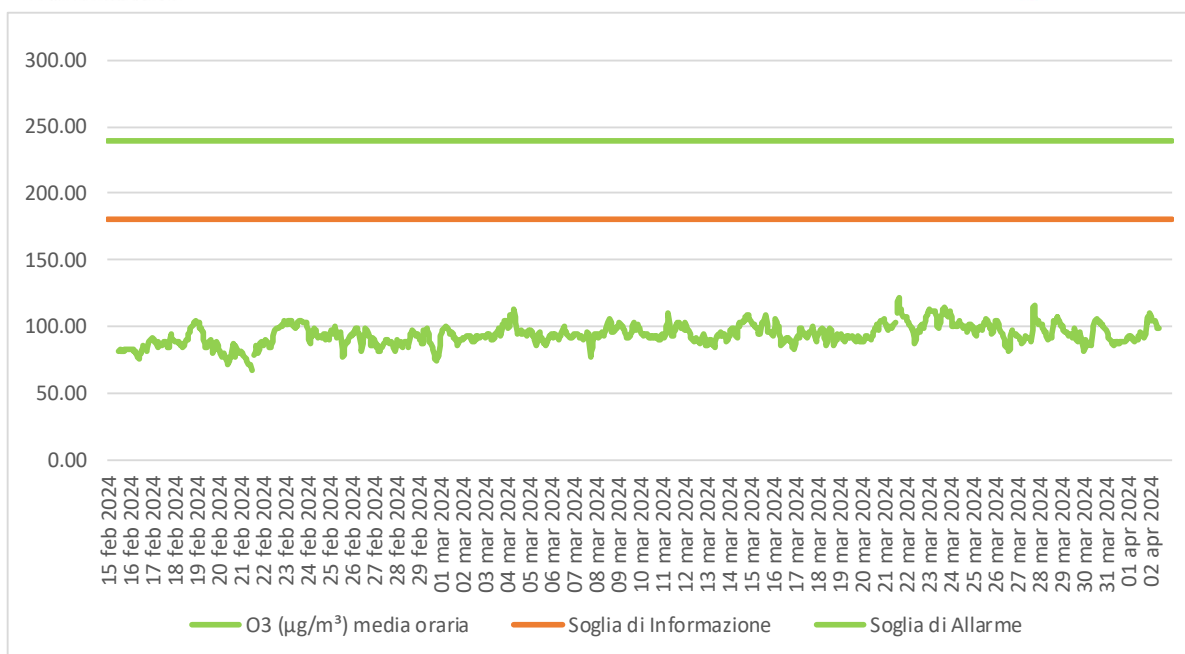
Figura 5.9 - Concentrazione (µg/m 3 ) media oraria di O 3 .
