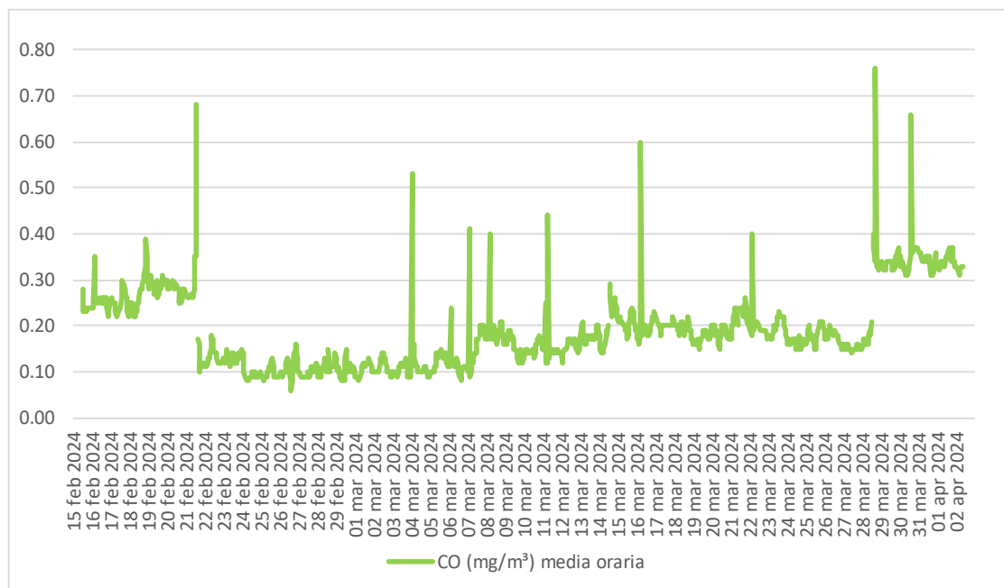
Figura 5.1 - Concentrazione (mg/m³) media oraria di CO.
