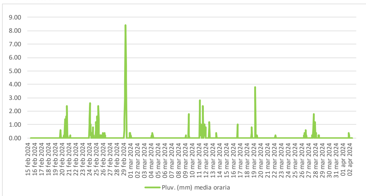
Figura 6.7 - Precipitazioni.
