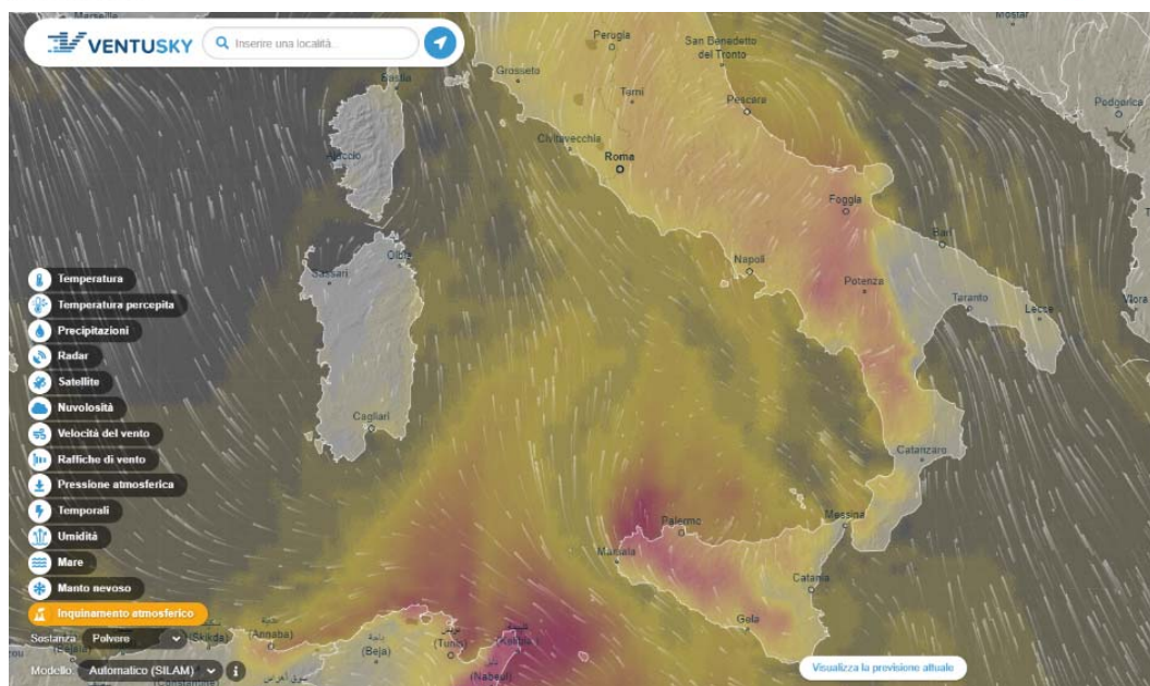
Figura 5.12 - Immagine modellistica del PM10 nel Mediterraneo per il giorno 31 Marzo 2024 ( https://www.ventusky.com )
