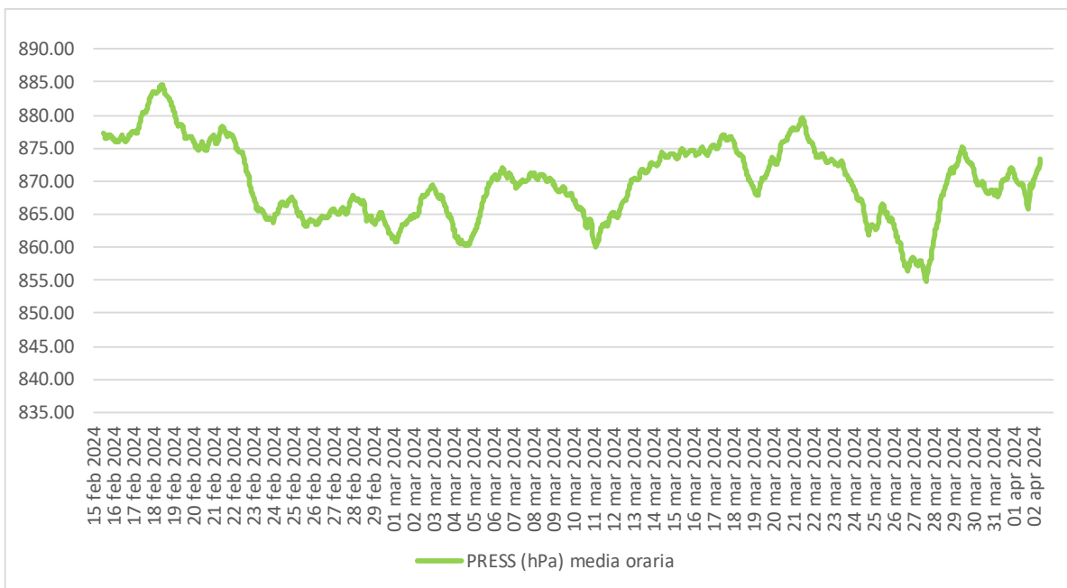
Figura 6.3 - Pressione atmosferica.
