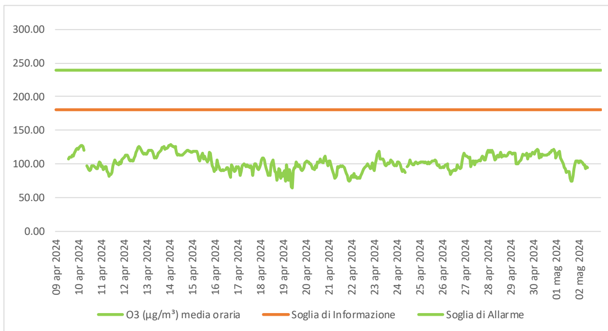
Figura 5.9 - Concentrazione ( \mu\text{g}/\text{m}^3 ) media oraria di \text{O}_3 .
