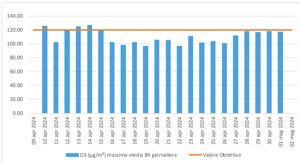
Figura 5.10 - Concentrazione ( \mu\text{g}/\text{m}^3 ) media mobile sulle 8 ore di \text{O}_3 .
