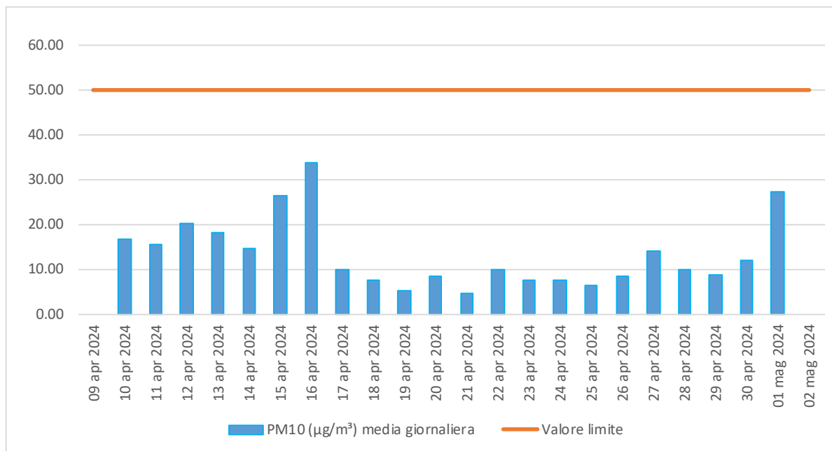
Figura 5.11 - Concentrazione (µg/m 3 ) media giornaliera di PM10.
