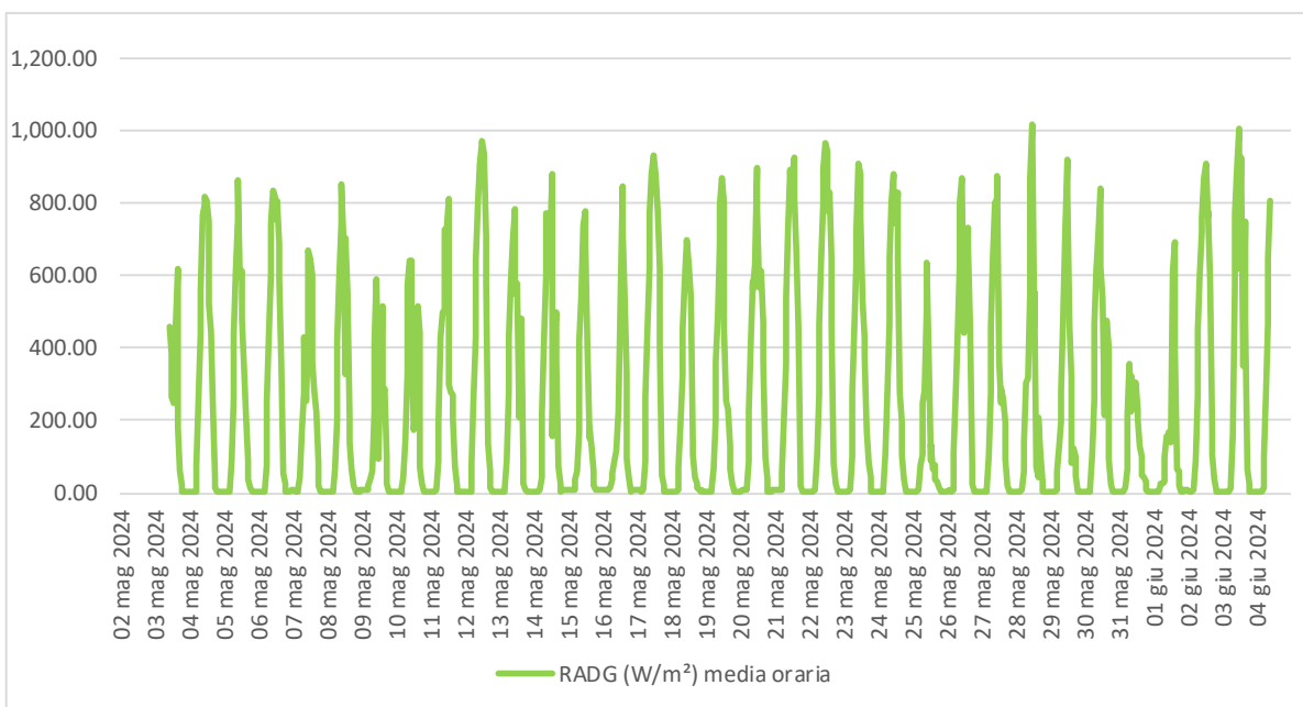
Figura 6.4 - Radiazione Solare.
