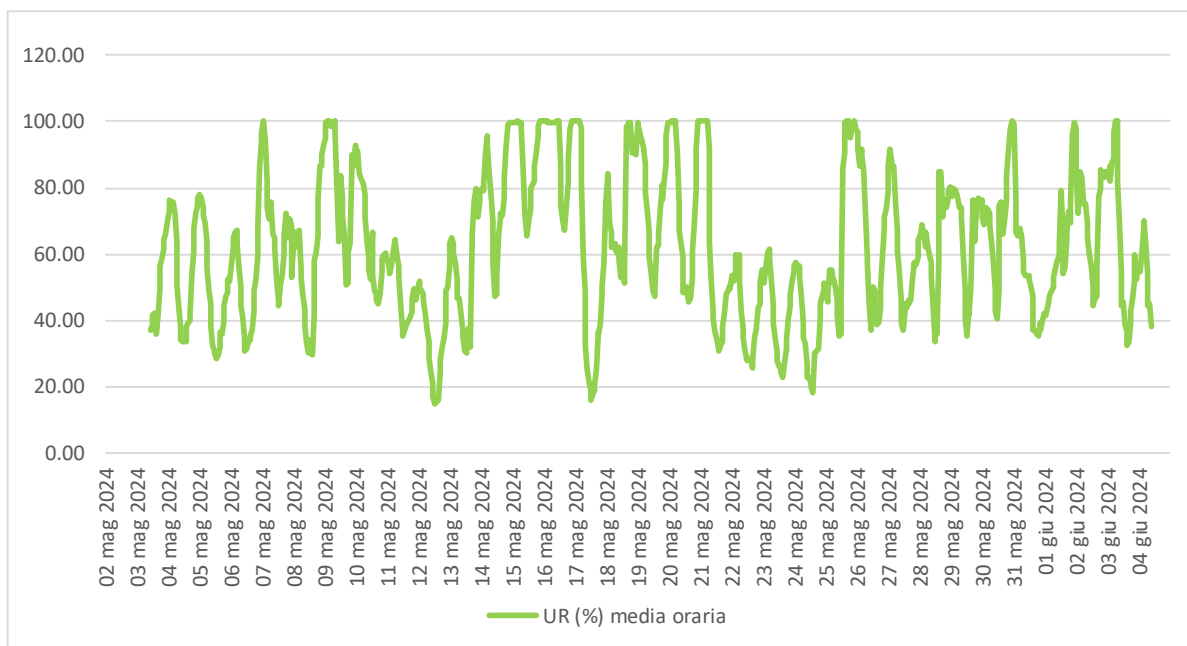
Figura 6.6 - Umidità Relativa.
