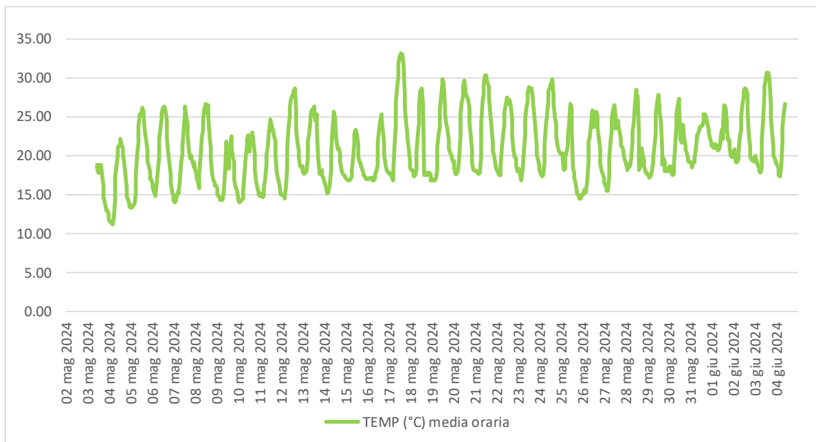
Figura 6.5 - Temperatura.
