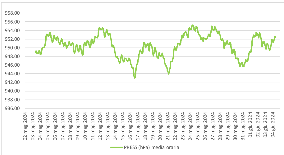
Figura 6.3 - Pressione atmosferica.
