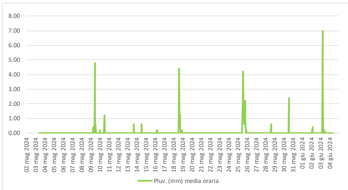
Figura 6.7 - Precipitazioni.
