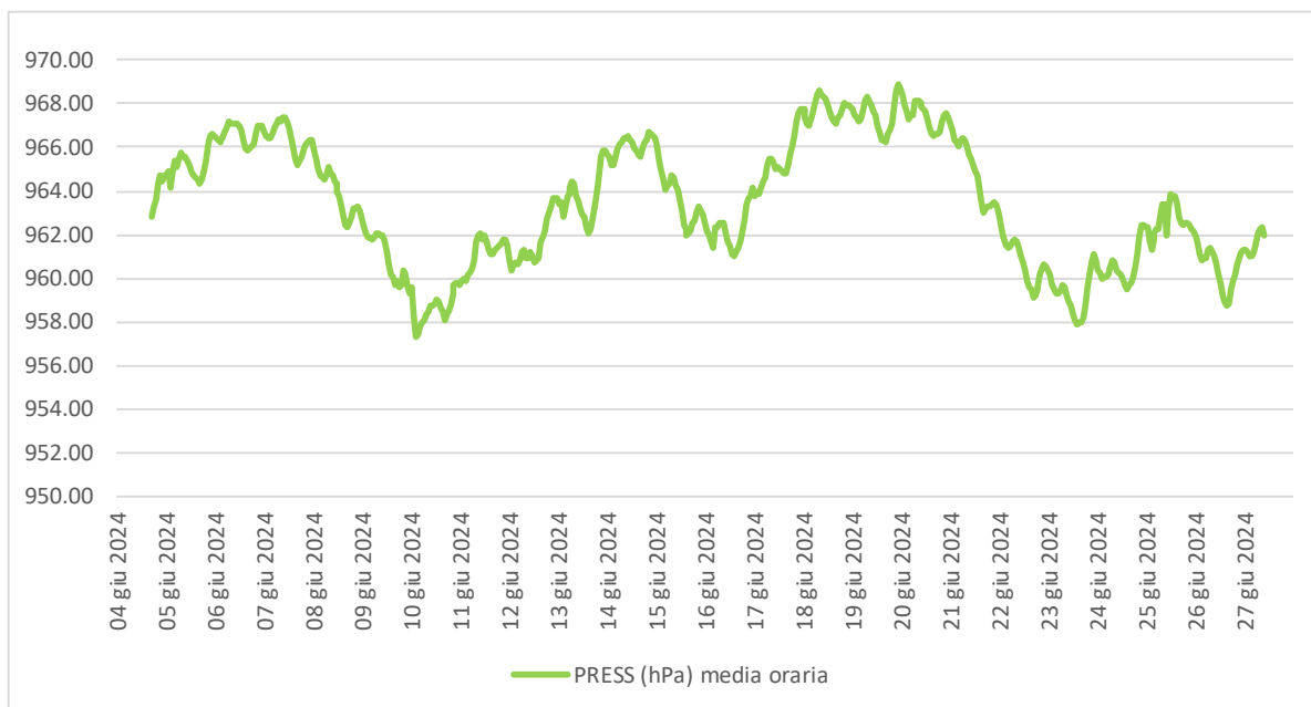
Figura 6.3 - Pressione atmosferica.
