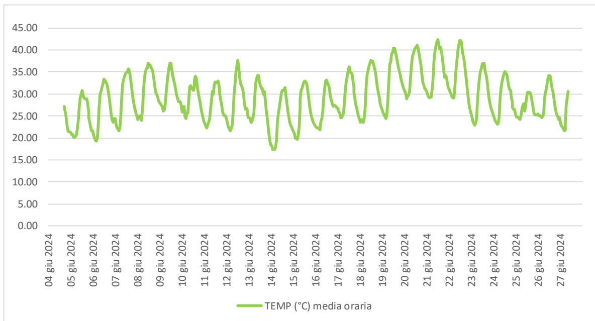
Figura 6.5 - Temperatura.
