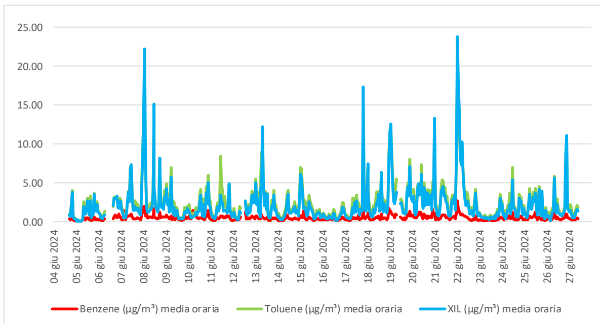
Figura 5.16 - Concentrazione ( \mu\text{g}/\text{m}^3 ) media oraria di BTX.
