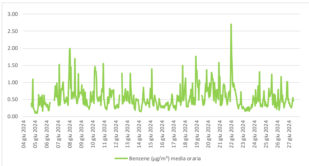
Figura 5.15 - Concentrazione ( \mu\text{g}/\text{m}^3 ) media oraria di Benzene.
