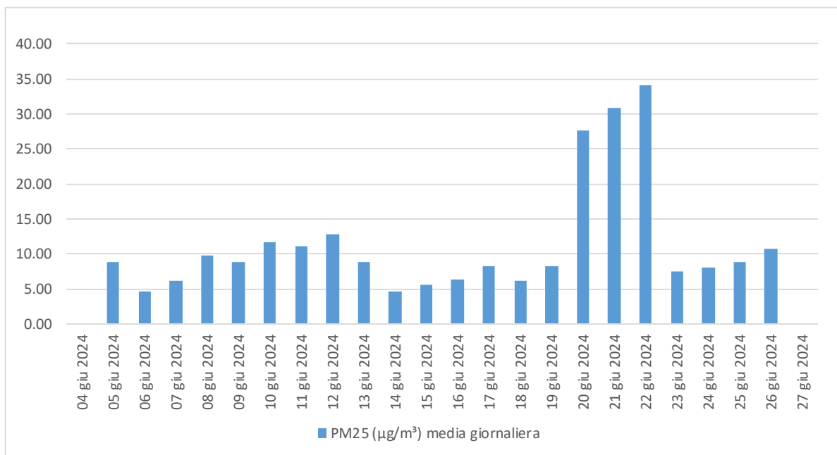
Figura 5.14 - Concentrazione (µg/m³) media giornaliera di PM2.5.
