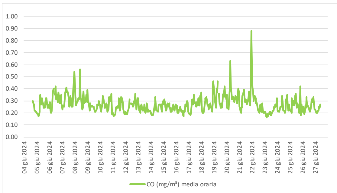
Figura 5.1 - Concentrazione (mg/m 3 ) media oraria di CO.
