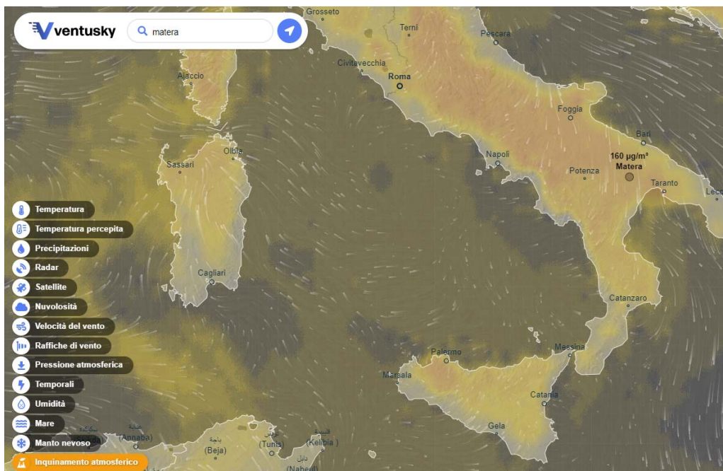
Figura 5.12 - Immagine modellistica del PM10 nel Mediterraneo per il giorno 20 Giugno 2024 ( https://www.ventusky.com )
