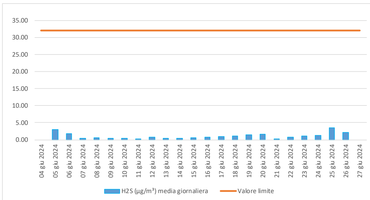
Figura 5.6 - Concentrazione ( \mu\text{g}/\text{m}^3 ) media giornaliera di H2S.
