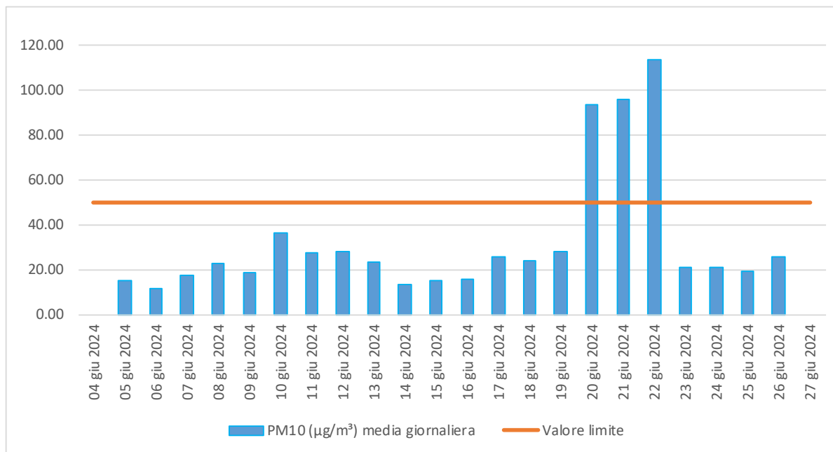
Figura 5.13 - Concentrazione (µg/m³) media giornaliera di PM10.
