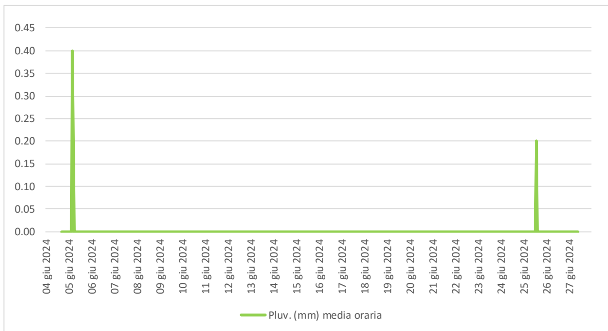
Figura 6.7 - Precipitazioni.
