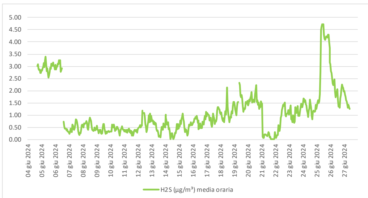
Figura 5.5 - Concentrazione ( \mu\text{g}/\text{m}^3 ) media oraria di H2S.
