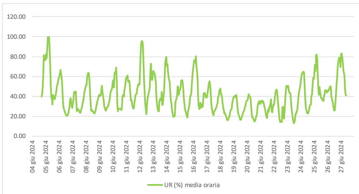
Figura 6.6 - Umidità Relativa.
