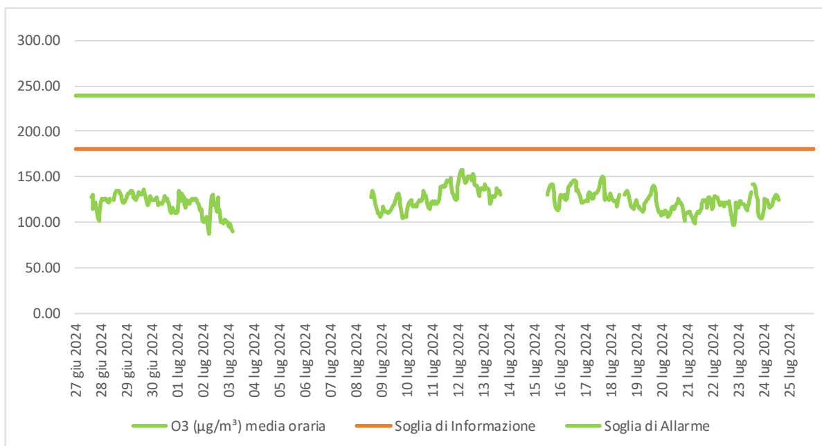
Figura 5.9 - Concentrazione ( \mu\text{g}/\text{m}^3 ) media oraria di O3.
