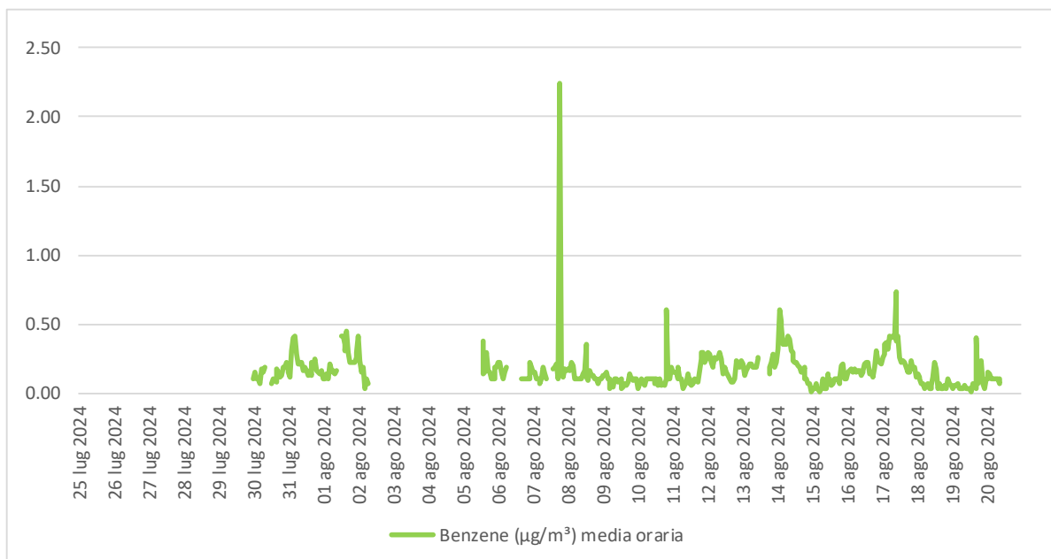
Figura 5.13 - Concentrazione ( \mu\text{g}/\text{m}^3 ) media oraria di Benzene.
