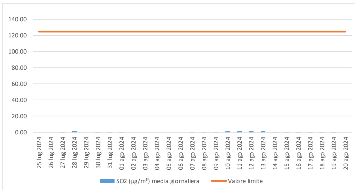
Figura 5.4 - Concentrazione (µg/m³) media giornaliera di SO 2 .
