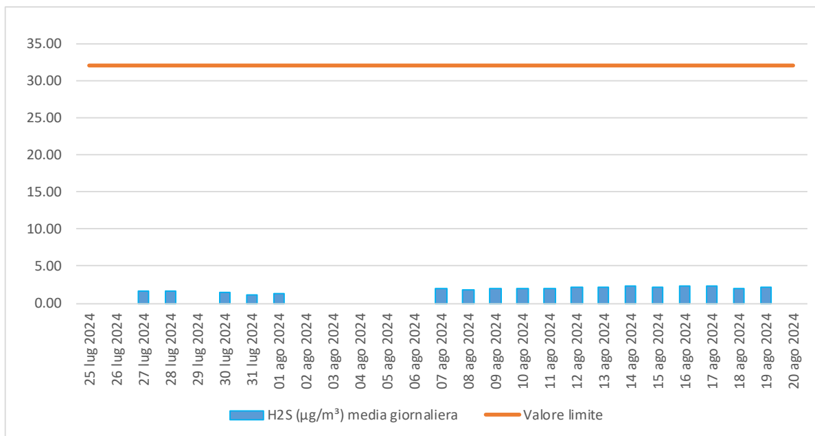
Figura 5.6 - Concentrazione (µg/m 3 ) media giornaliera di H 2 S.
