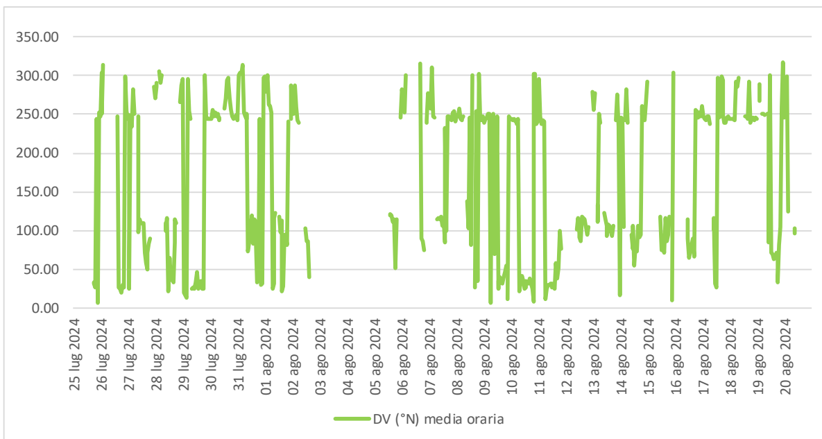
Figura 6.2 - Direzione del vento.
