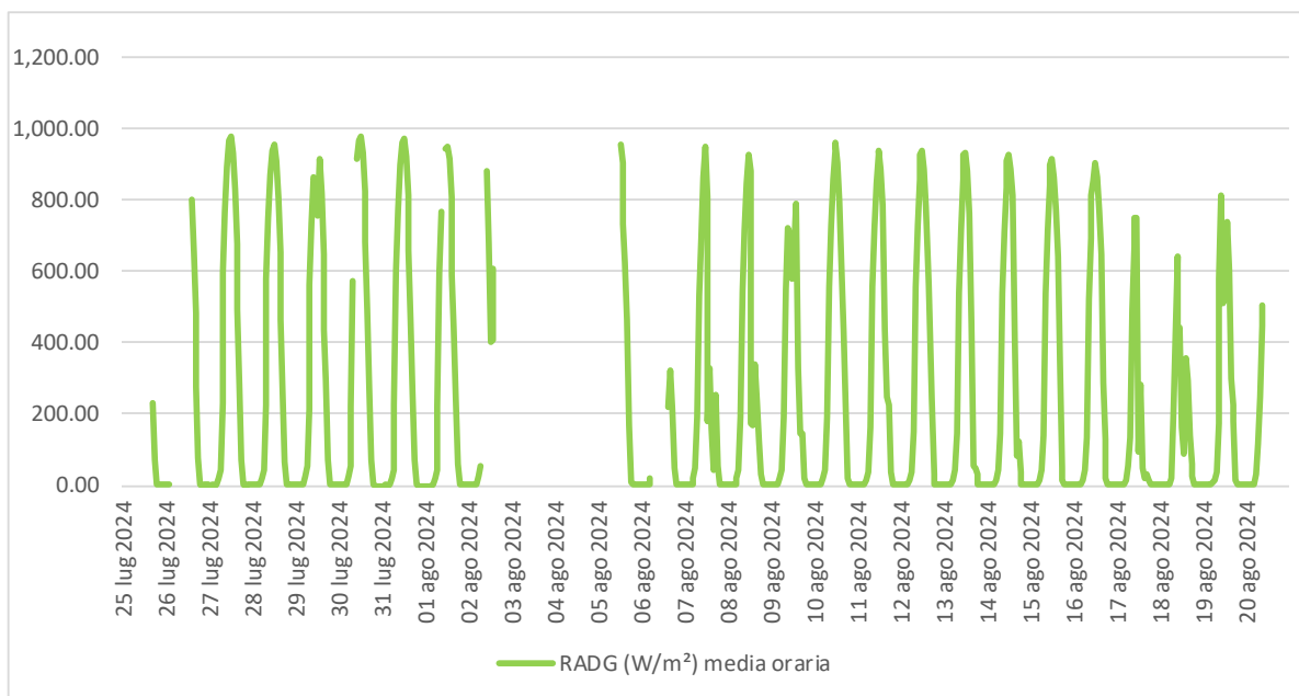
Figura 6.4 - Radiazione Solare.
