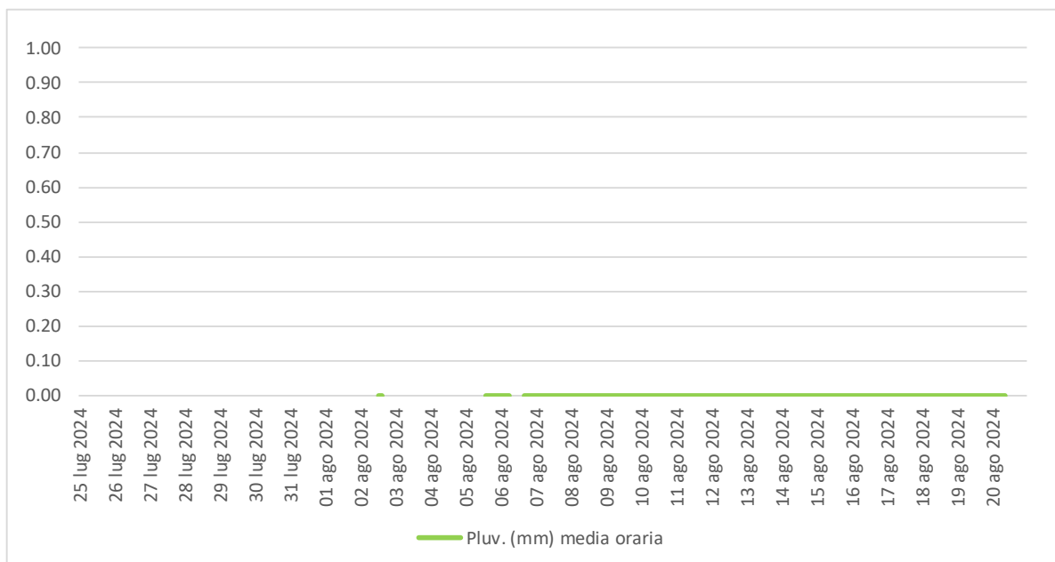
Figura 6.7 - Precipitazioni.
