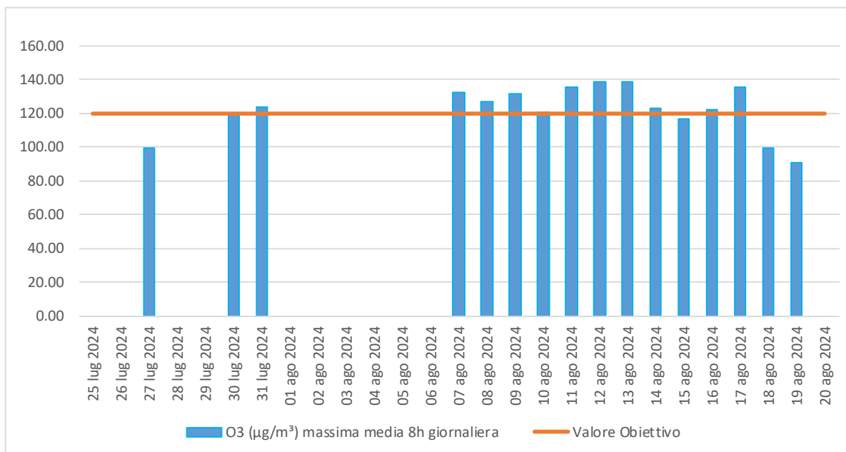
Figura 5.10 - Concentrazione ( \mu\text{g}/\text{m}^3 ) media mobile sulle 8 ore di \text{O}_3 .
