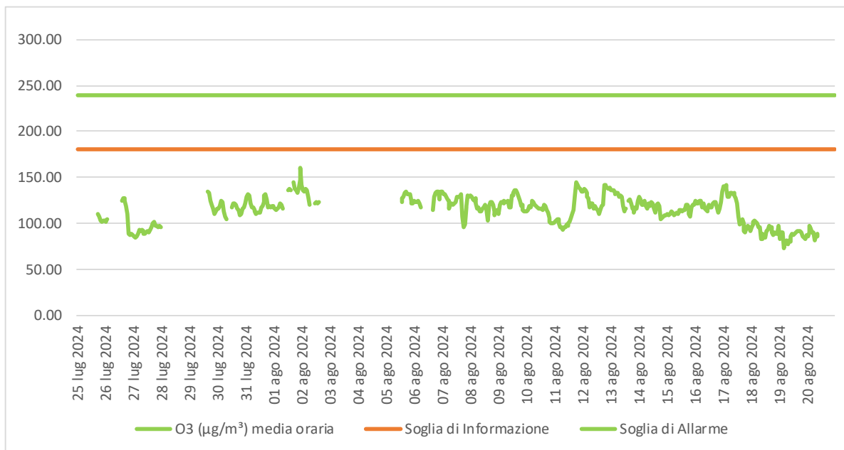
Figura 5.9 - Concentrazione ( \mu\text{g}/\text{m}^3 ) media oraria di \text{O}_3 .
