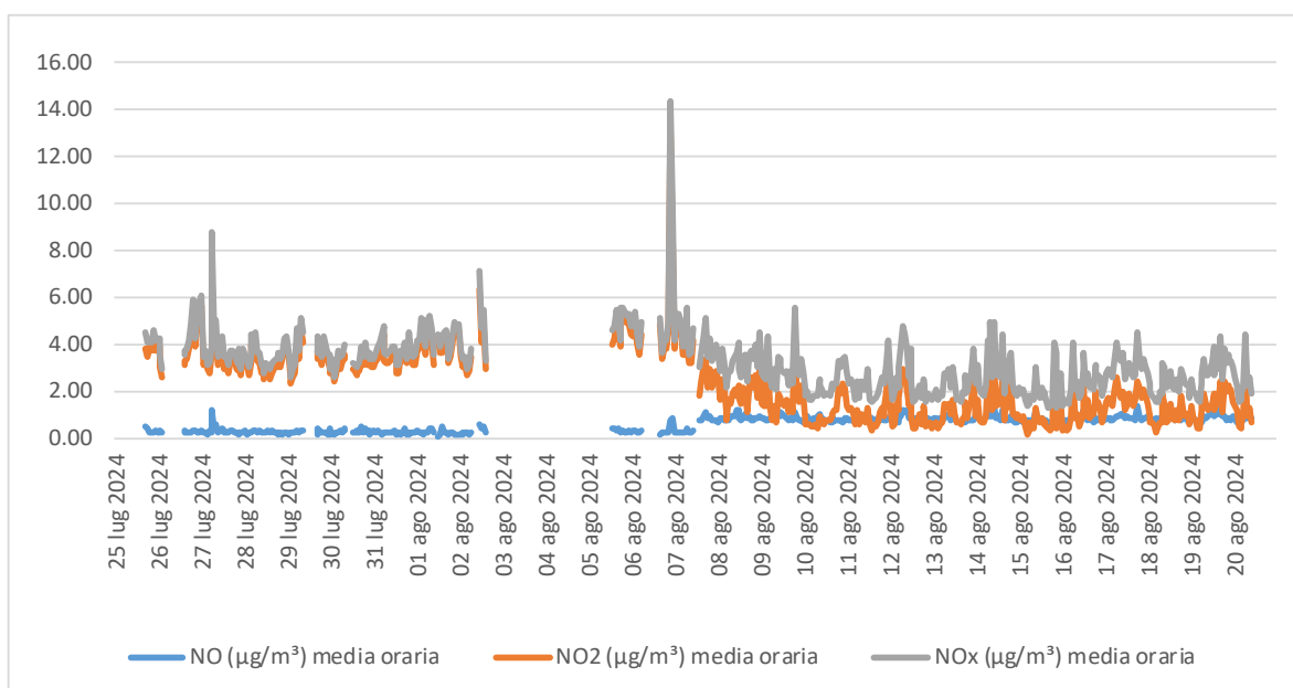
Figura 5.8 - Concentrazione ( \mu\text{g}/\text{m}^3 ) media oraria di Ossidi di Azoto.
