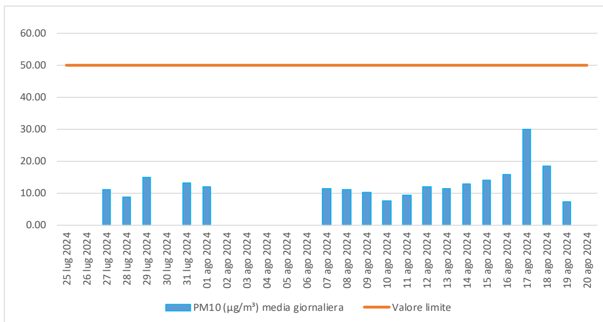
Figura 5.11 - Concentrazione ( \mu\text{g}/\text{m}^3 ) media giornaliera di PM10.
