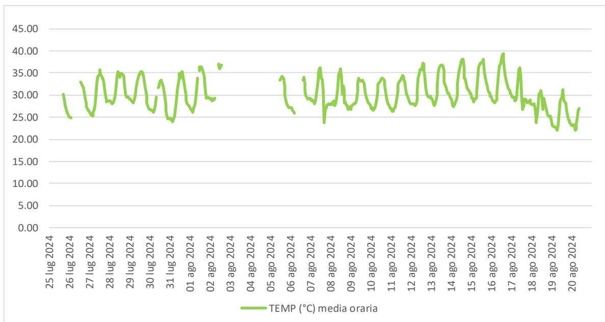
Figura 6.5 - Temperatura.
