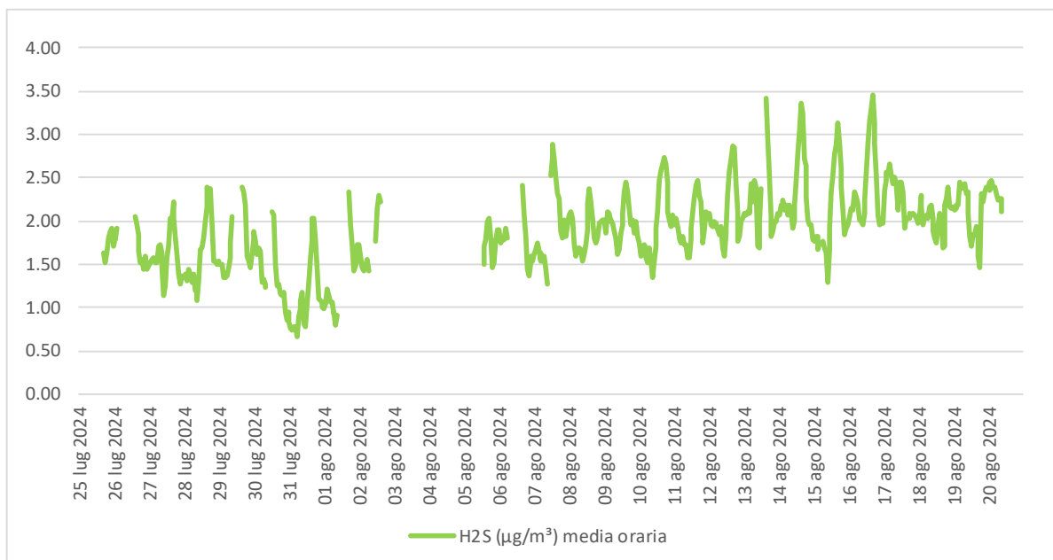
Figura 5.5 - Concentrazione (µg/m 3 ) media oraria di H 2 S.
