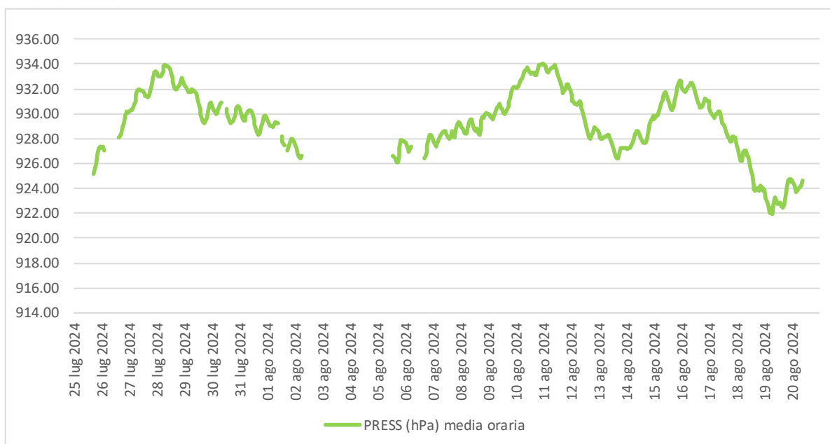
Figura 6.3 - Pressione atmosferica.
