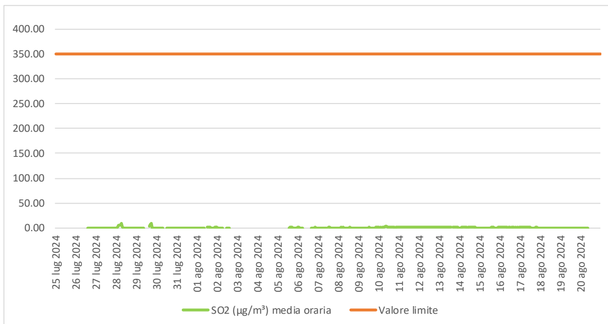
Figura 5.3 - Concentrazione (µg/m³) media oraria di SO 2 .
