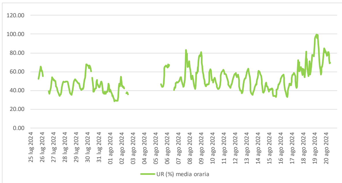
Figura 6.6 - Umidità Relativa.
