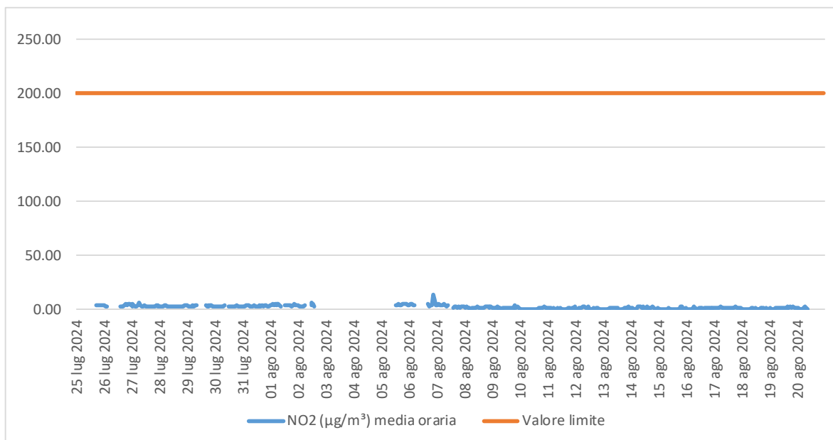
Figura 5.7 - Concentrazione ( \mu\text{g}/\text{m}^3 ) media oraria di \text{NO}_2 .
