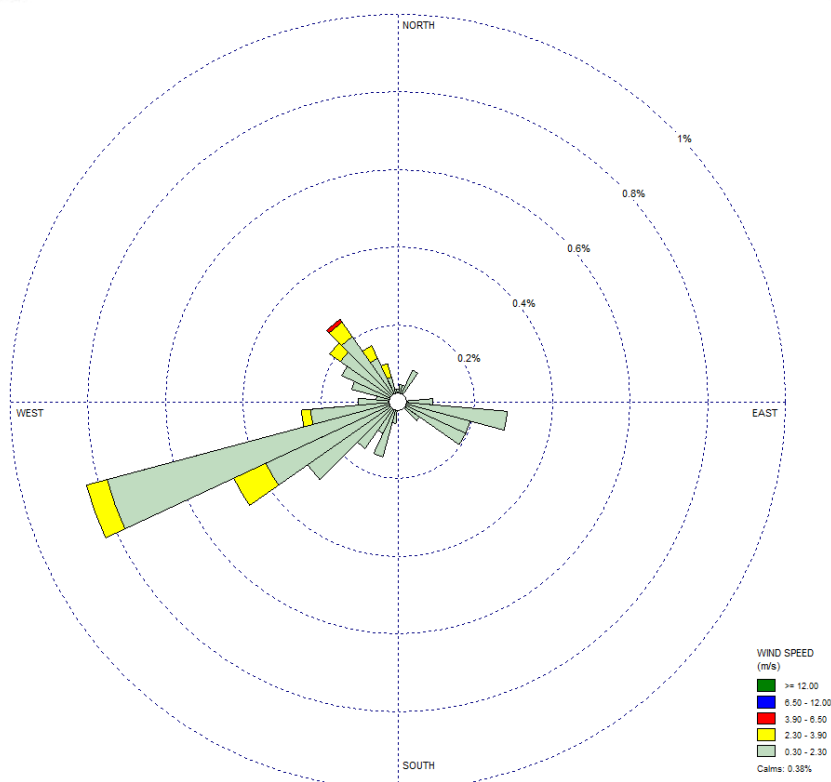
Figura 6.9 - Rosa dei venti - Media del periodo.
