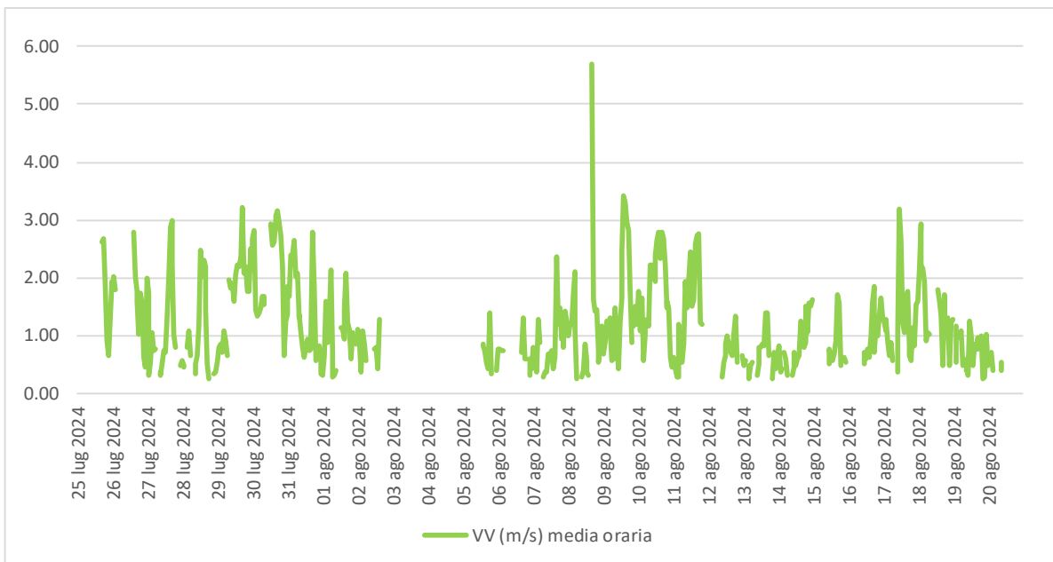
Figura 6.1 - Velocità del vento.
