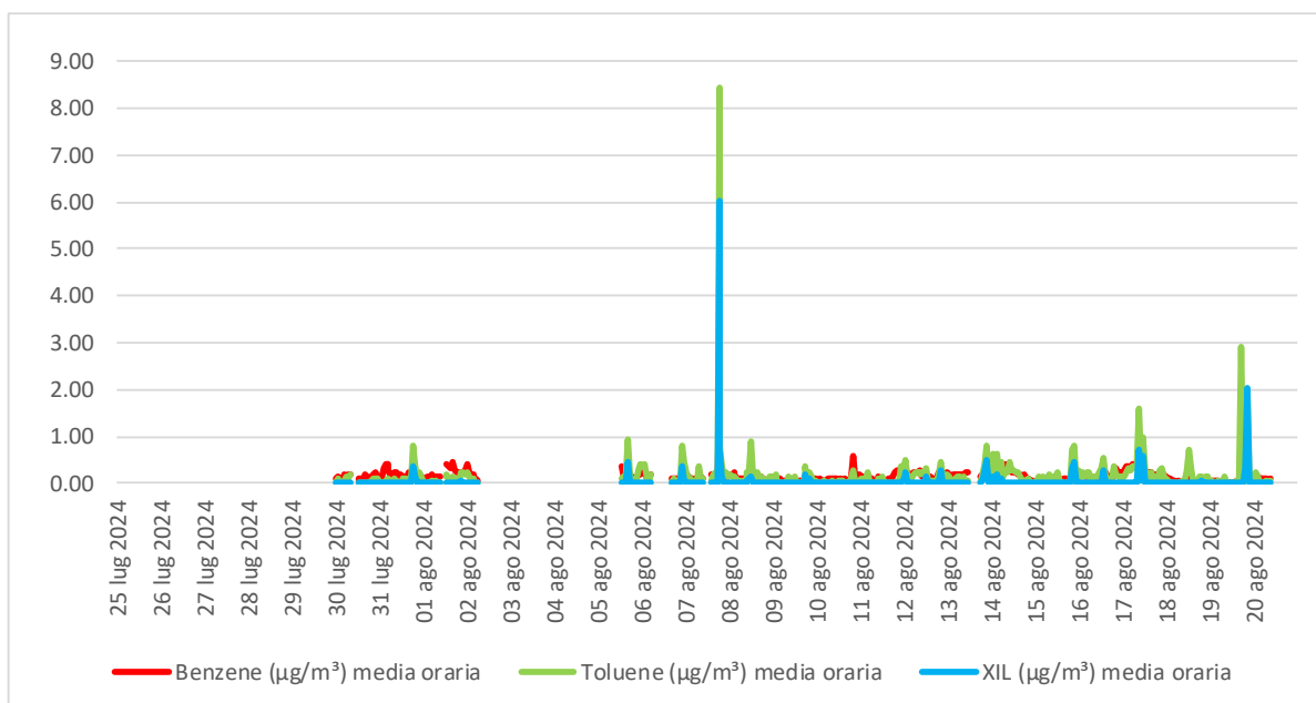
Figura 5.14 - Concentrazione ( \mu\text{g}/\text{m}^3 ) media oraria di BTX.
