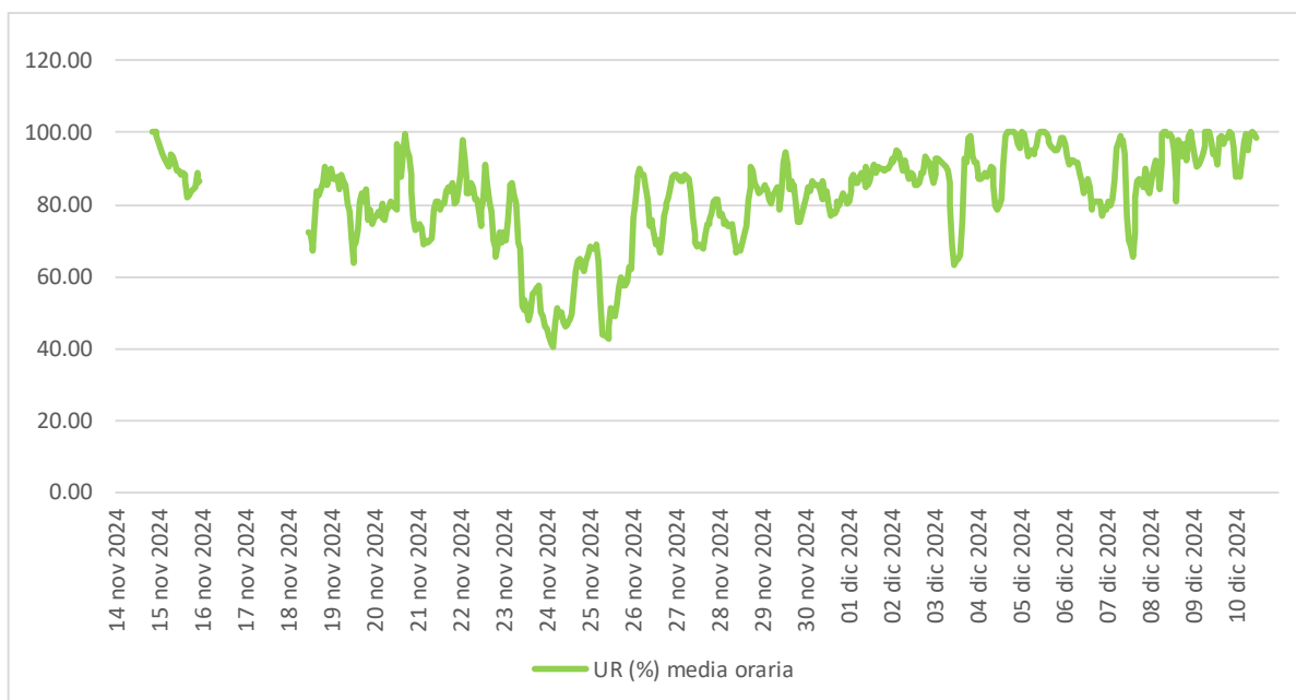
Figura 6.6 - Umidità Relativa.
