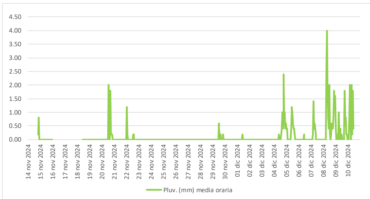
Figura 6.7 - Precipitazioni.
