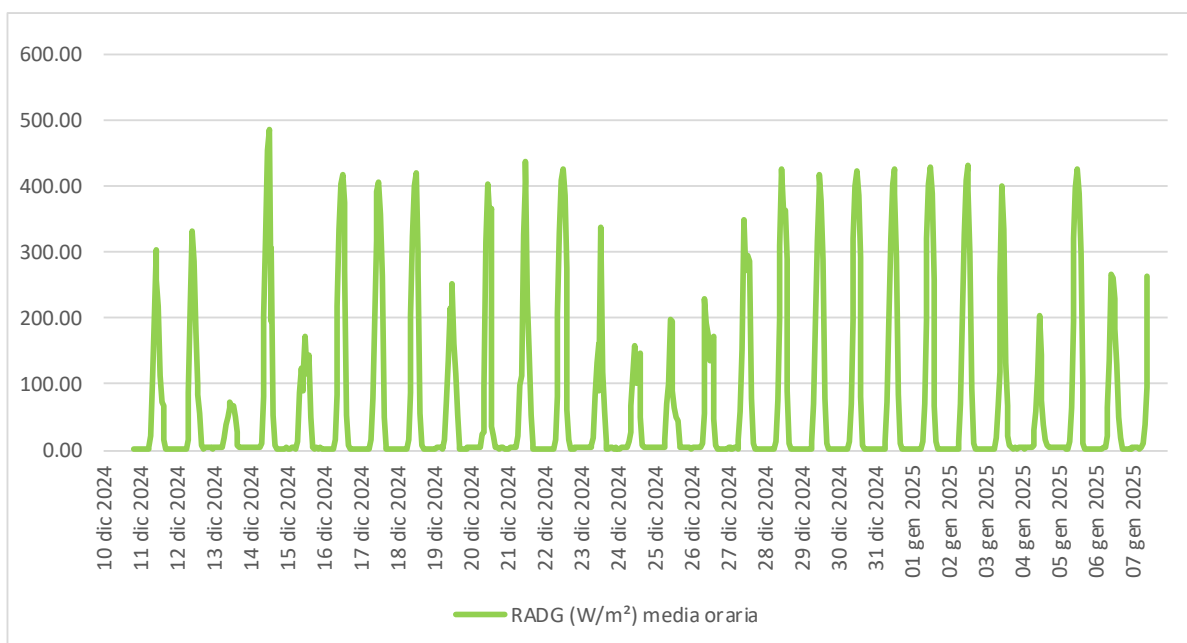
Figura 6.4 - Radiazione Solare.
