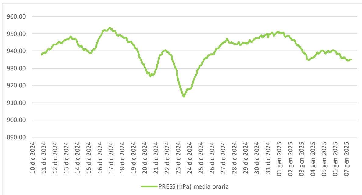
Figura 6.3 - Pressione atmosferica.
