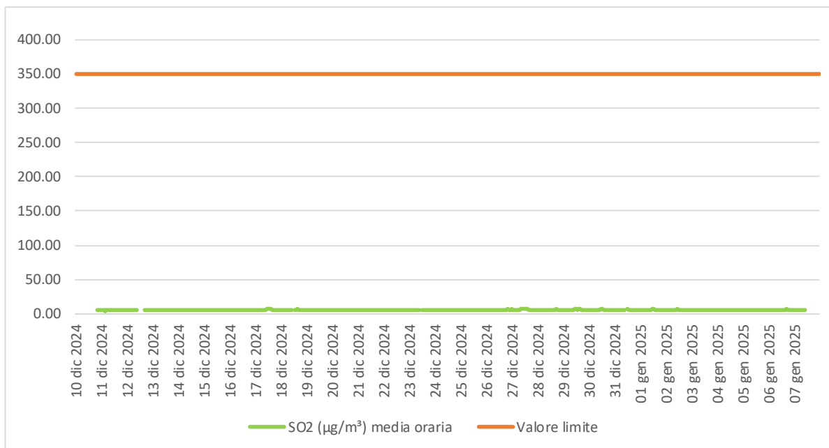
Figura 5.3 - Concentrazione (µg/m³) media oraria di SO 2 .
