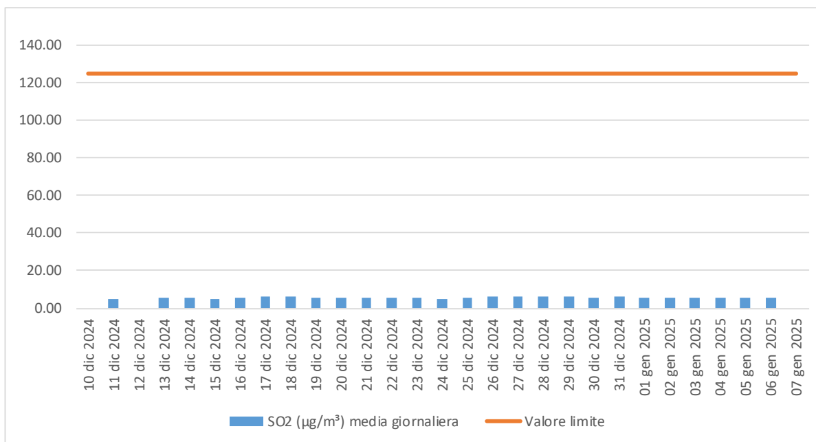
Figura 5.4 - Concentrazione (µg/m³) media giornaliera di SO 2 .
