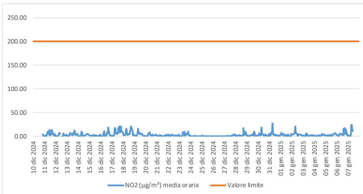
Figura 5.7 - Concentrazione (µg/m 3 ) media oraria di NO 2 .
