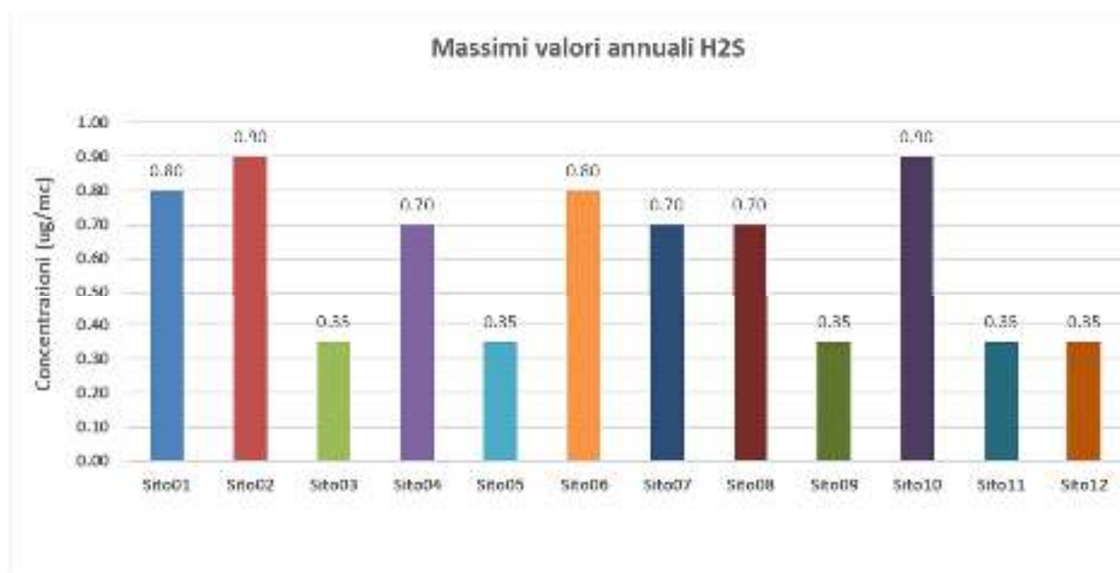
Figura 5.13 - Grafico dei valori massimi di concentrazione di H 2 S rilevati - Anno 2024.
