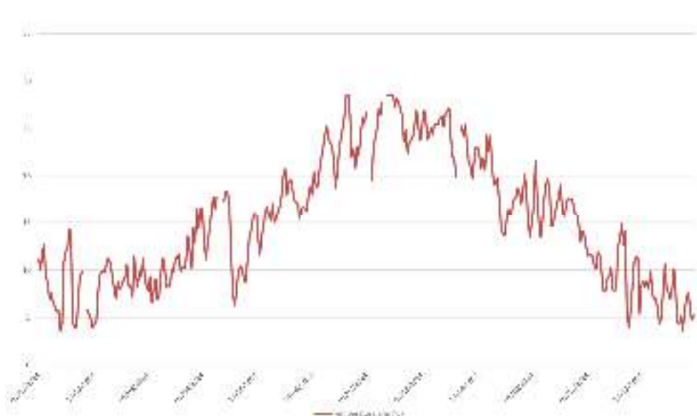
Figura 6.1 - Andamento della Temperatura nel periodo di riferimento - Stazione di Viggiano.
