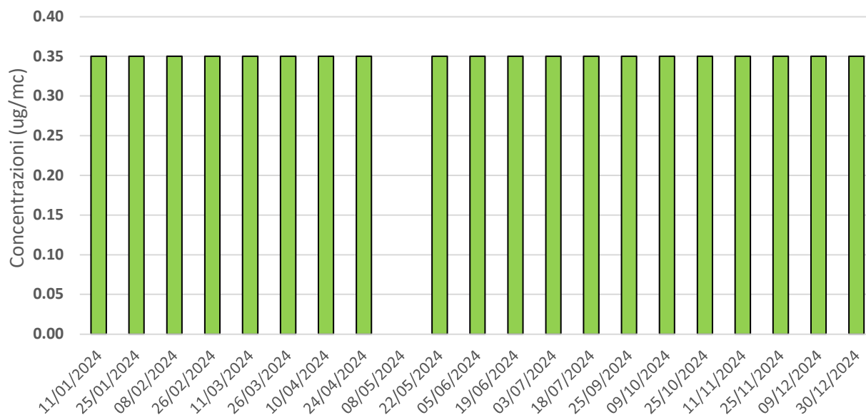
Figura 5.3 - Sito 03 - Grafico dei valori di concentrazione di H 2 S rilevati.
