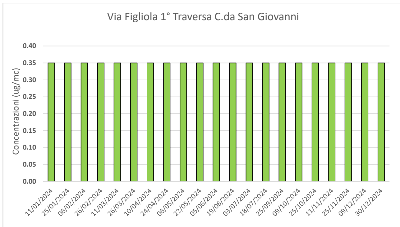
Figura 5.11 - Sito 11 - Grafico dei valori di concentrazione di H 2 S rilevati.
