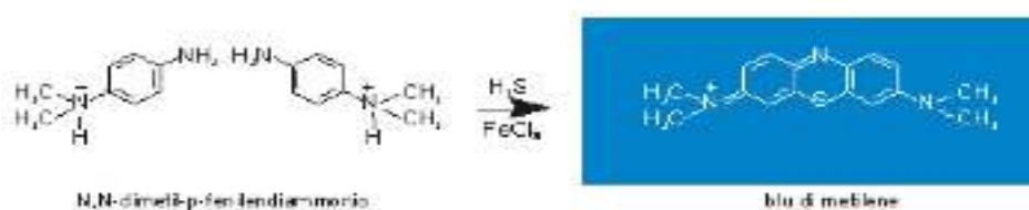
Figura 4.13 - Schema di chemiadsorbimento dell'H 2 S.
