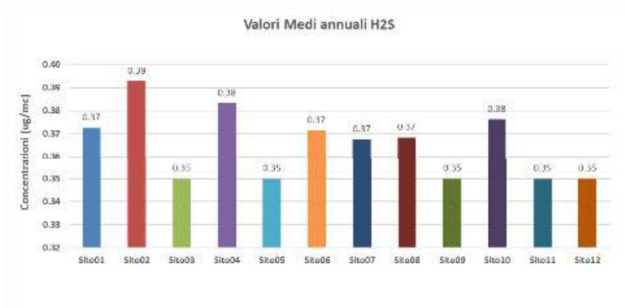
Figura 5.14 - Grafico dei valori medi di concentrazione di H 2 S rilevati - Anno 2024.
