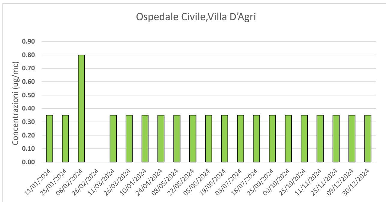
Figura 5.1 - Sito 01 - Grafico dei valori di concentrazione di H 2 S rilevati.
